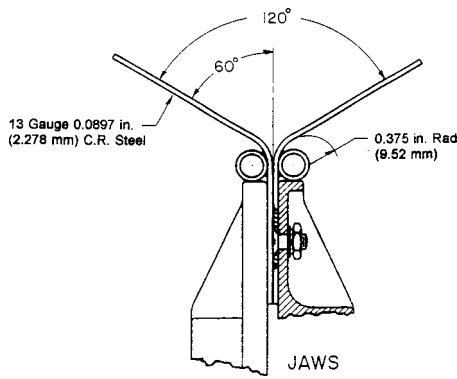
FIG. 30 Flexure Tester
