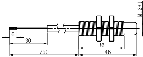
开关组件 Switch Assembly
