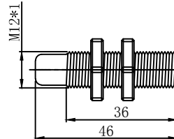
磁铁组件 Magnet Assembly
