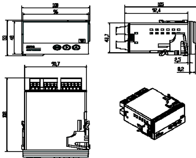
图 1 ZW160X 系列仪表安装尺寸图
