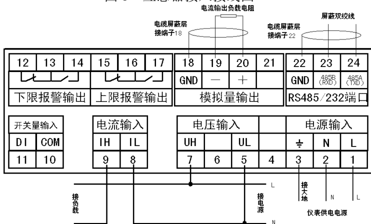
图 6 普通接线图
