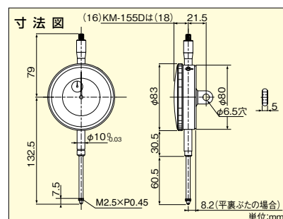
KM-155D ストローク50mmの 中二針タイプ 目量0.01mm 測定範囲50mm ・ショックブルーフ
