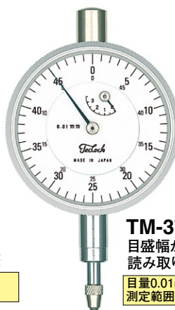
TM-36 0.005mmの 左右振分目盛 目量0.005mm 測定範囲3.5mm
