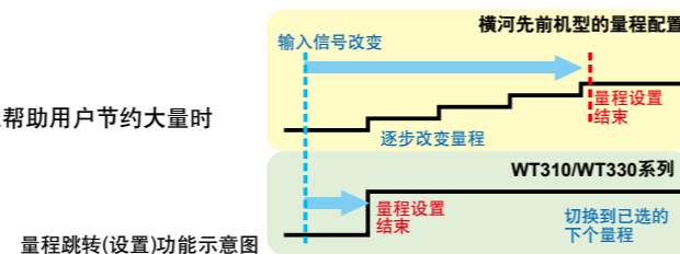
量程跳转(设置)功能示意图
