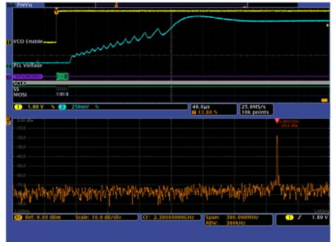
图 4 – 在 VCO 启用后大约 340 \mu s 时，VCO/PLL 终于稳定在正确频率 2.400 GHz 上。
