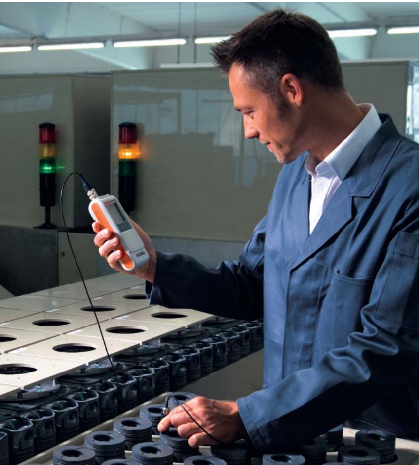
使用FTA3.3H 探头对刚生产出来的引擎活塞进行质量检测。
