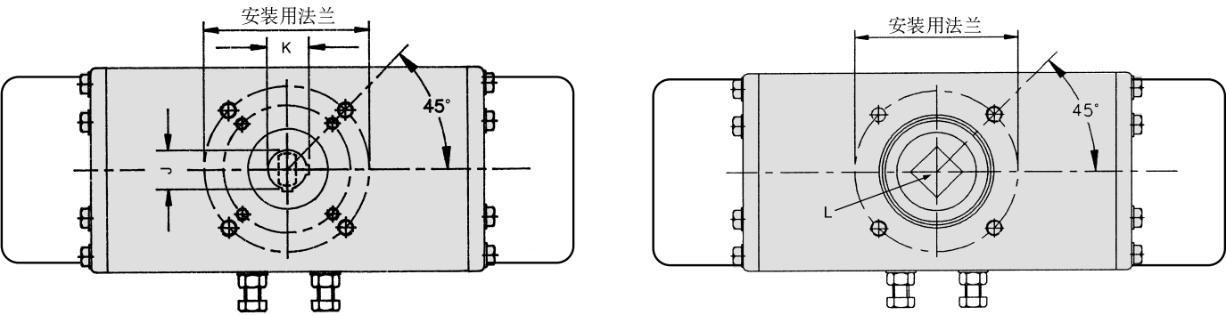
执行机构齿轮轴底部的驱动详图
