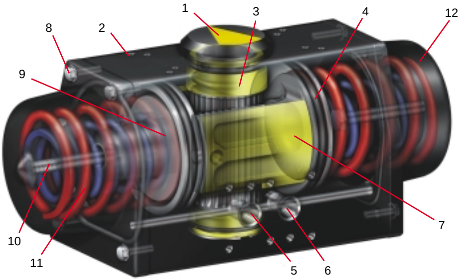
型号 002-036 的典型视图 (仅作参考, 弹簧颜色可能不同)
