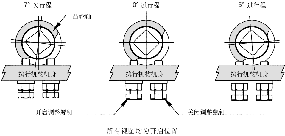
Namur 附属接合器细节 (图 79D)
