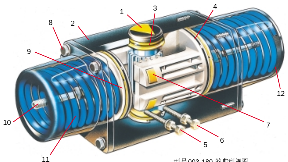
型号 003-180 的典型视图 (型号 002 不带行程限位器)
