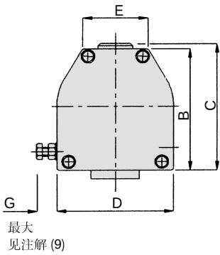
外形图 79U/E - 型号 065, 090 和 180
