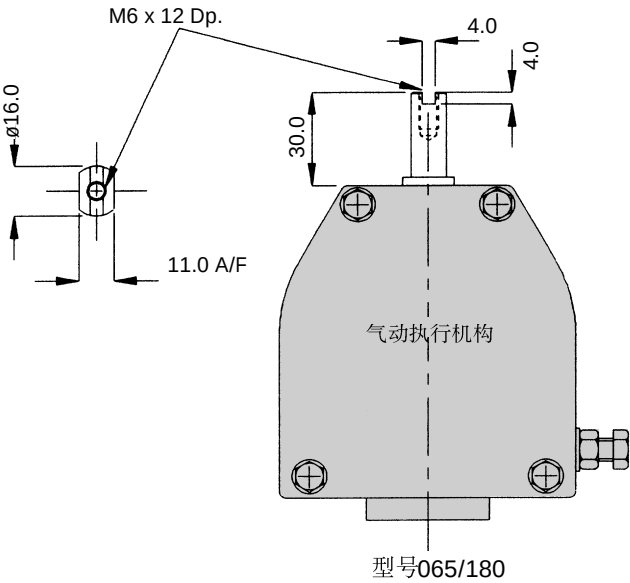
Namur 附属接合器细节 (图 79D)
