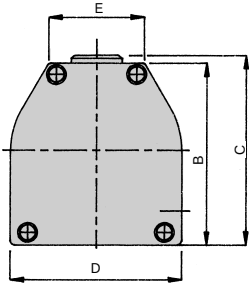
外形图 79D - 型号 002 至 018
