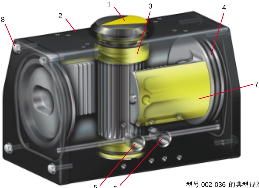
型号 002-036 的典型视图
