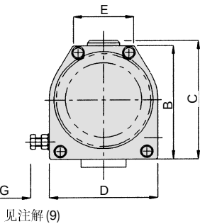
外形图 79U/E - 型号 065S, 090S 和 180S
