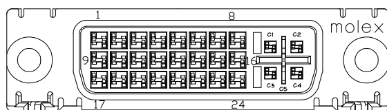
DVI-D 接口
