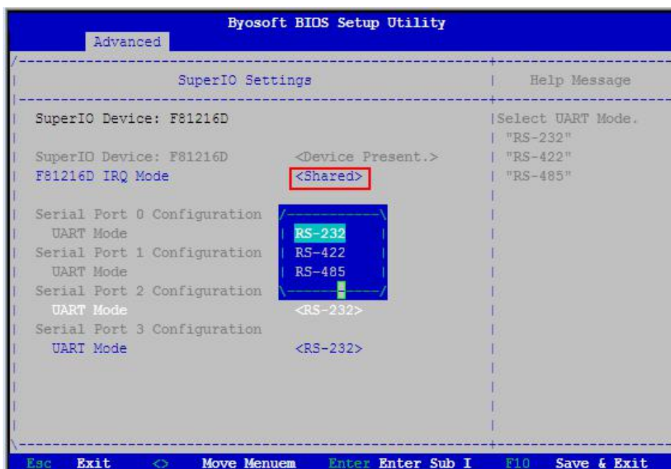
图 5 Super IO 配置页面
