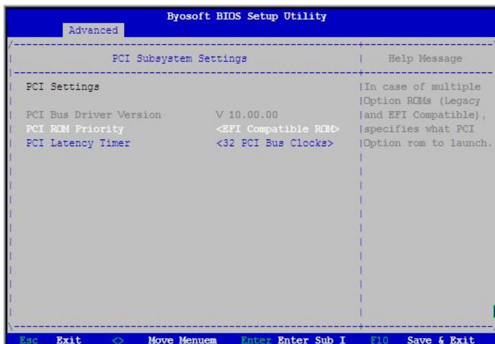
图 8 PCI 配置页面
