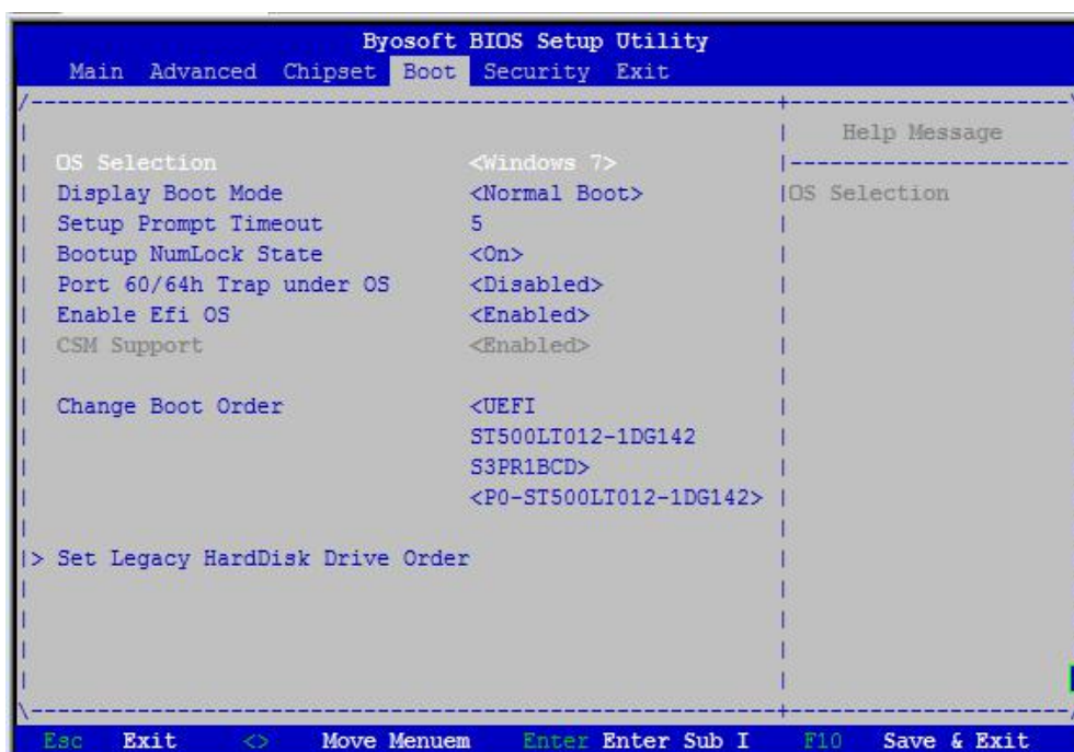
图 13 启动设备配置页面
