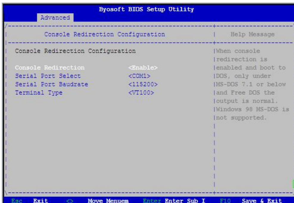
图 9 Console 配置页面
