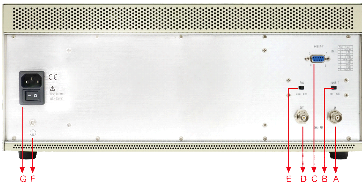
图3 PXIeC-7318C 后面板
