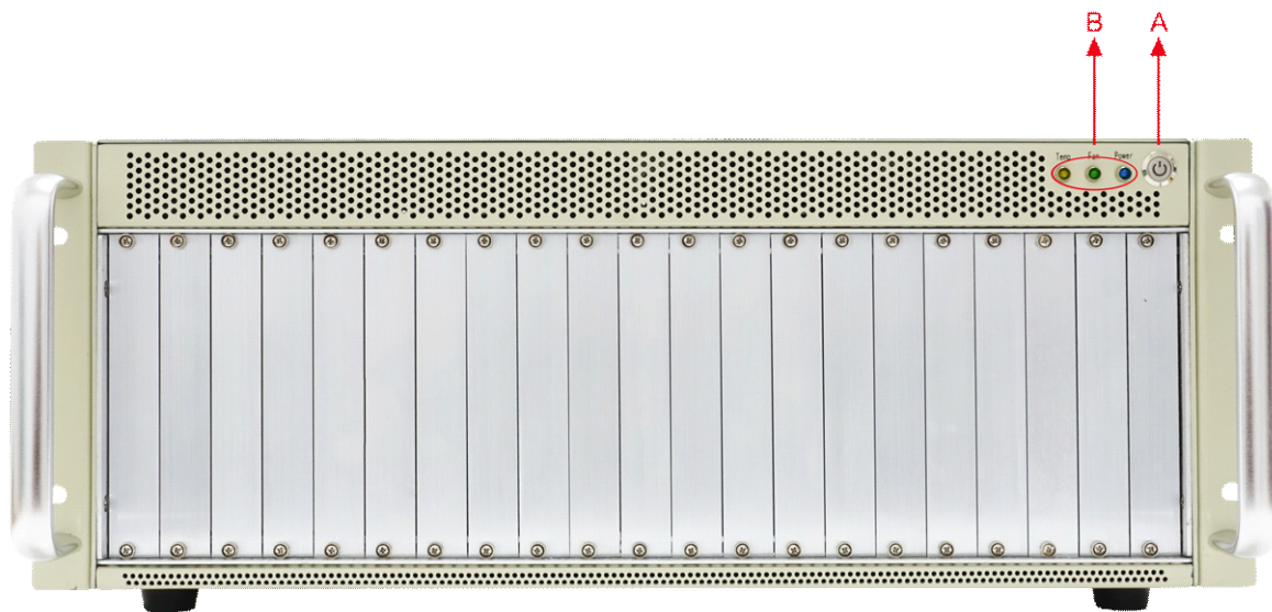
图 1 前面板图
