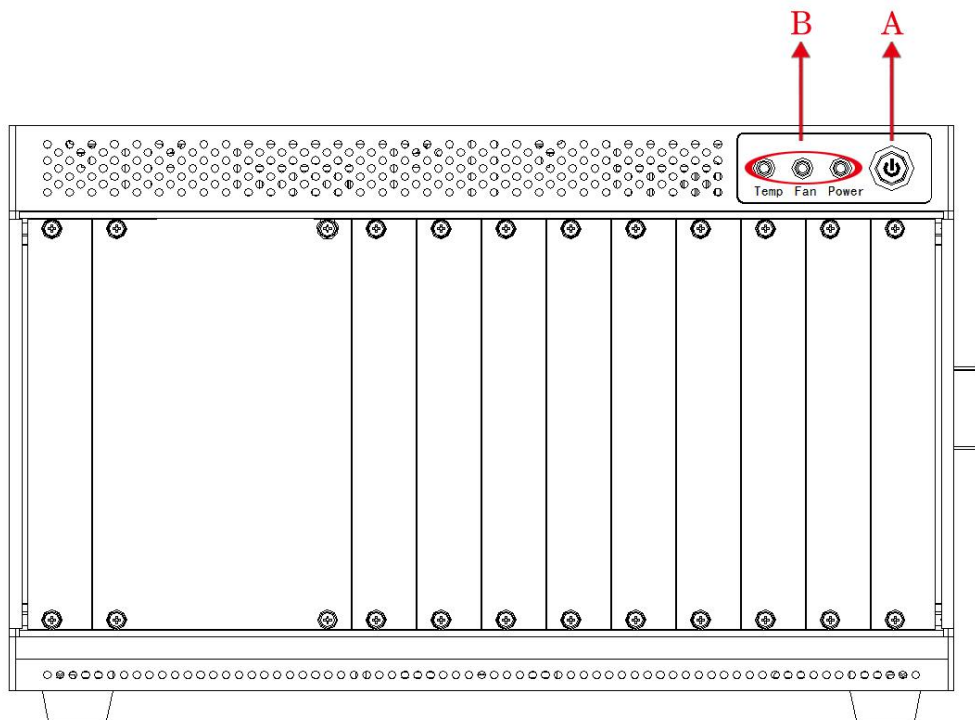
图 2-6 前面板图
