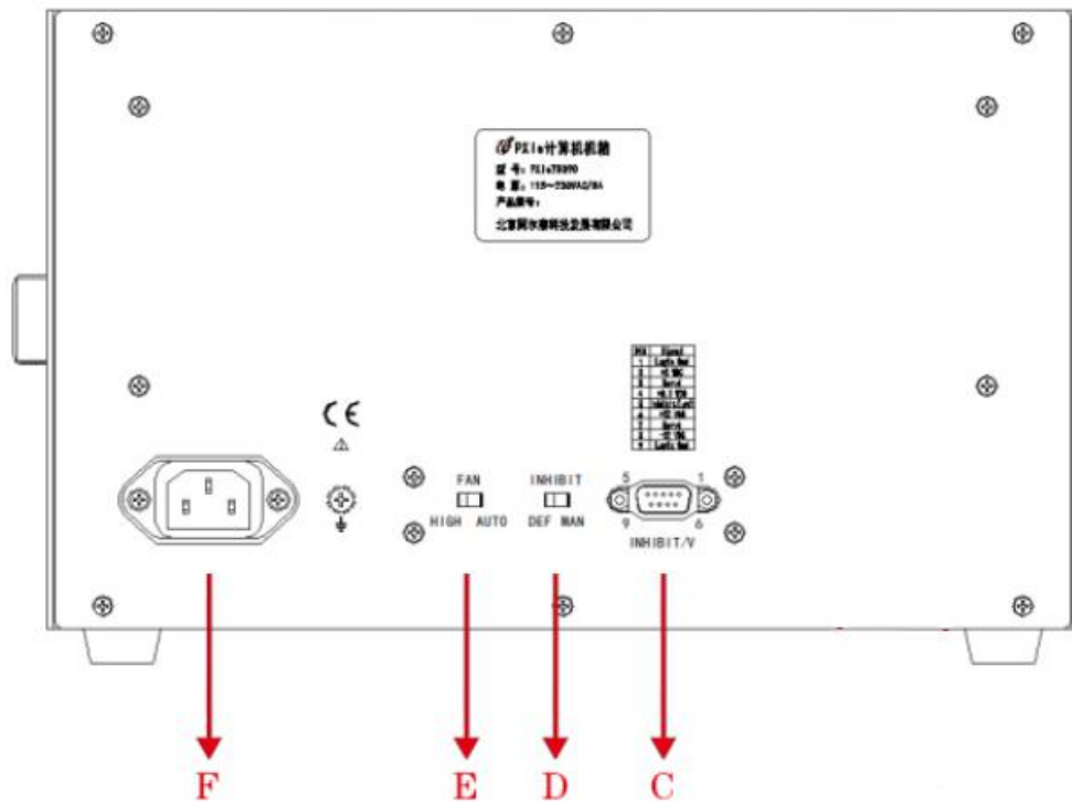
图 2-7: PXIeC-7309L 后面板
