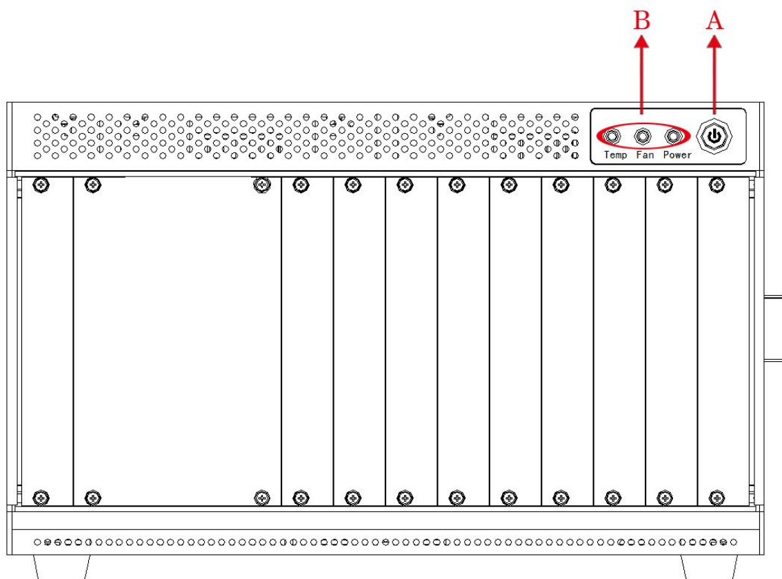
图 2-6 前面板图
