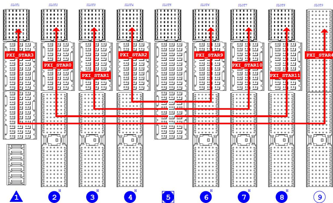
图 2-10 单端星形触发
