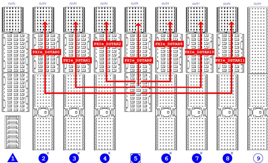
图 2-11 差分星形触发
