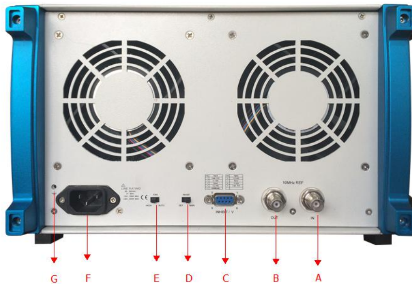
图 2-7: PXIeC-7309 后面板
