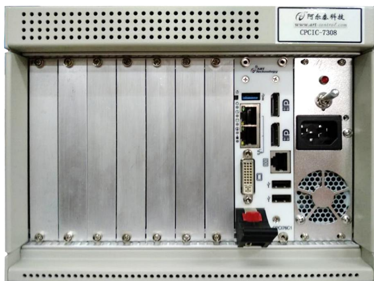
图 1-1 CPCIC-7308 正视图
