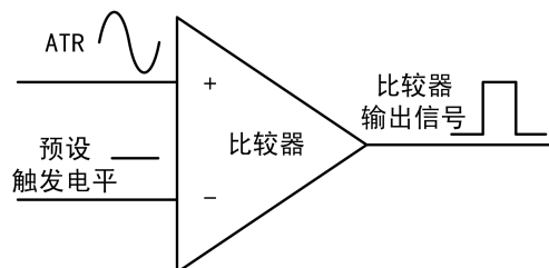
图4-9-4 比较器
