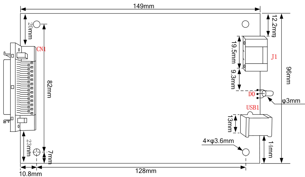
图 3-2-1 USB2894 板卡尺寸图
