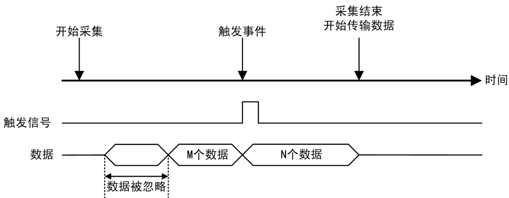
图 4-10-2 中间触发
