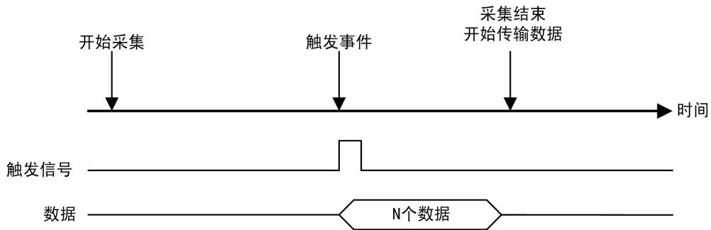
图 4-10-3 后触发
