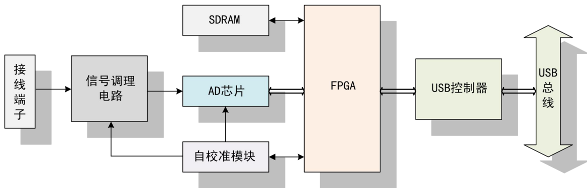
图 2-2-1 USB2894 系统框图
