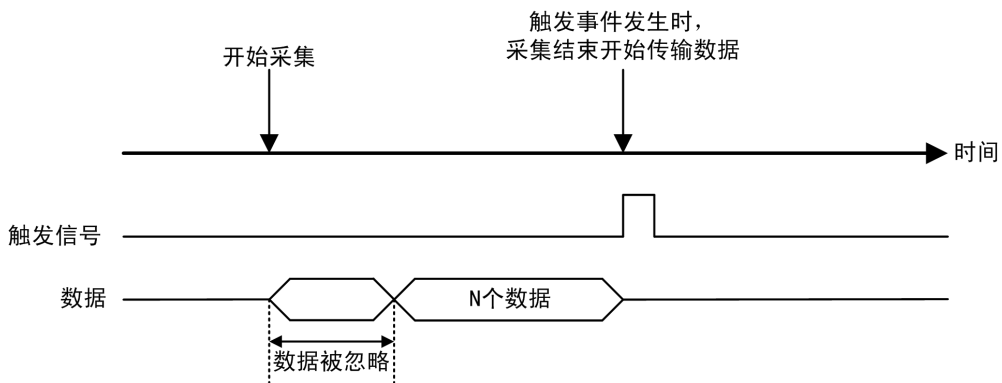
图 4-10-4 预触发
