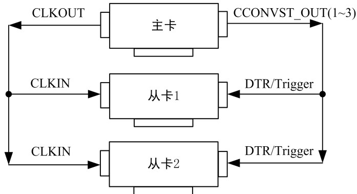
图 4-11-1 主从卡级联
