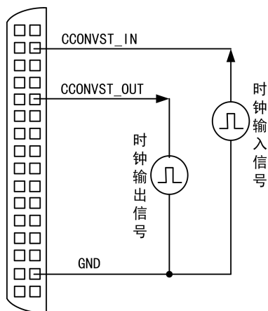
图 4-7-1 时钟输入输出的连接
