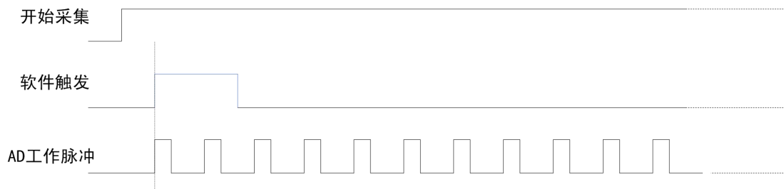
图4-9-3 AD内触发
