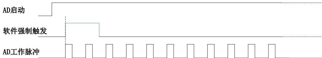
图4-9-3 AD内触发
