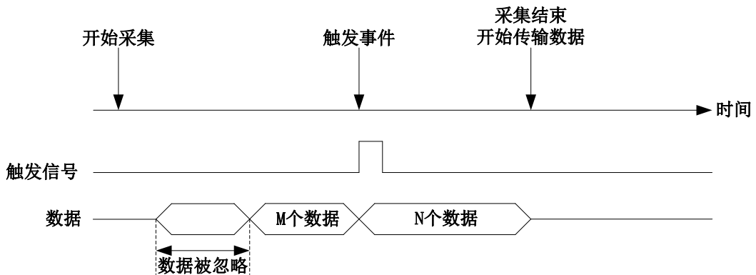
图 4-10-2 中间触发
