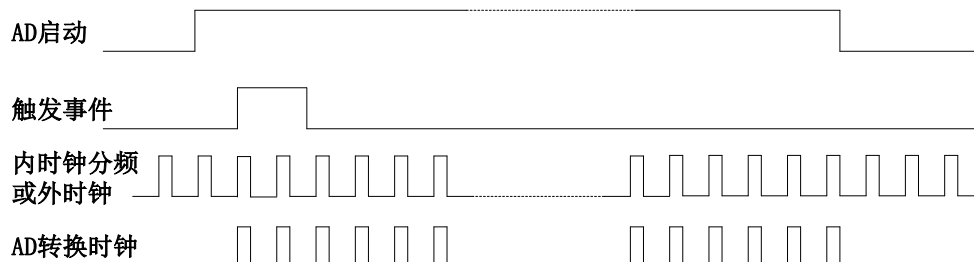
图4-8-1 AD采集
