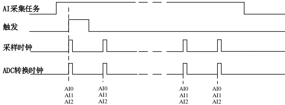
图4-6-3 连续采样
