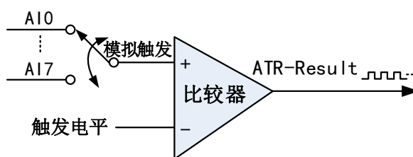
图4-8-7 比较器
