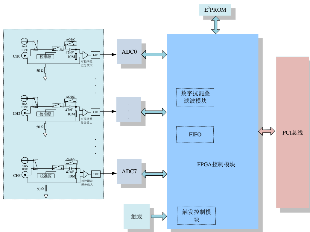
图 2.2.1 USB8814 系统框图
