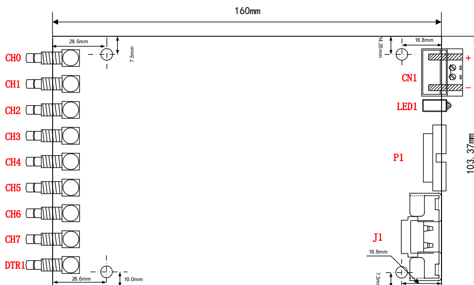
图 3-2-1 板卡尺寸图
