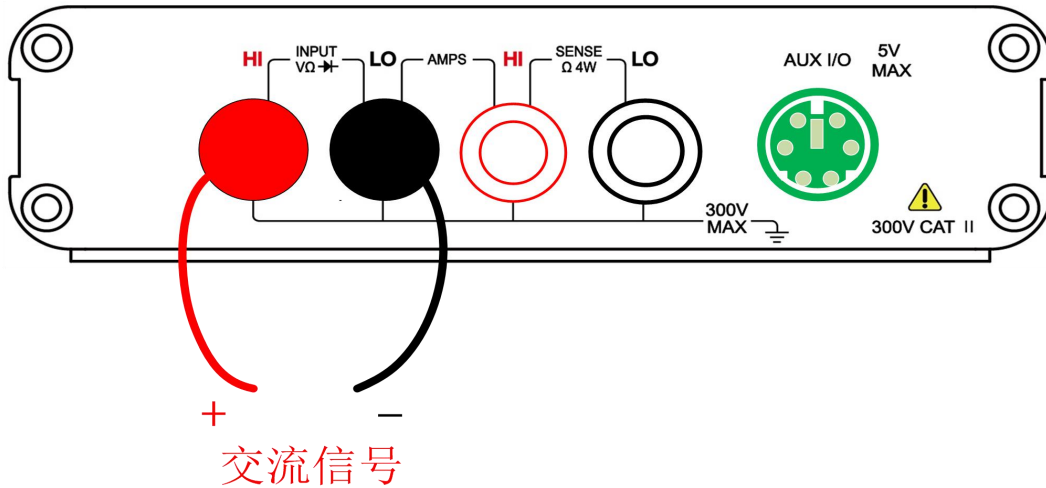
图 3-3 测量逻辑频率接线方式
