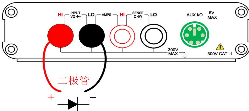
图 3-4 二极管测量接线方式
