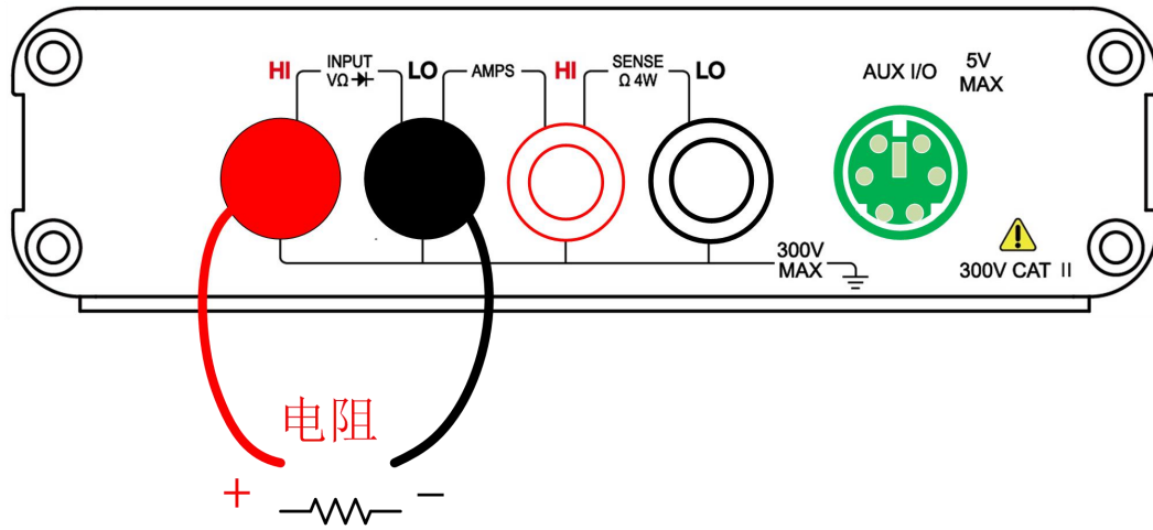
图 3-6 2W 电阻测量接线方式
