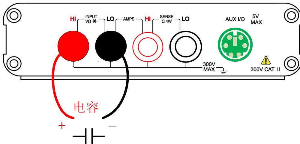
图 3-5 测量电容接线方式
