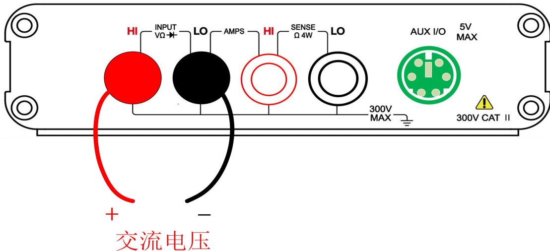
图 3-1-1 测量交流电压接线方式
