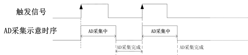
图 3-10-1 触发时序示意图
