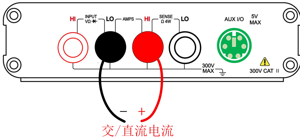
图 3-8 测量交、直流电流接线方式
