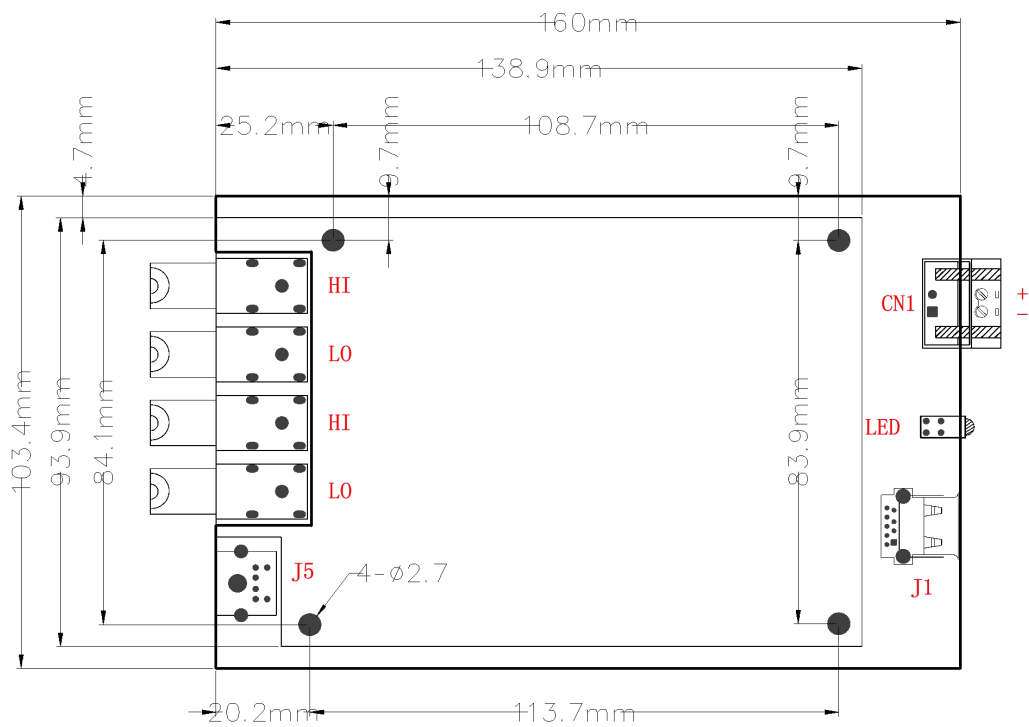
图 2-2-1 板卡尺寸图
