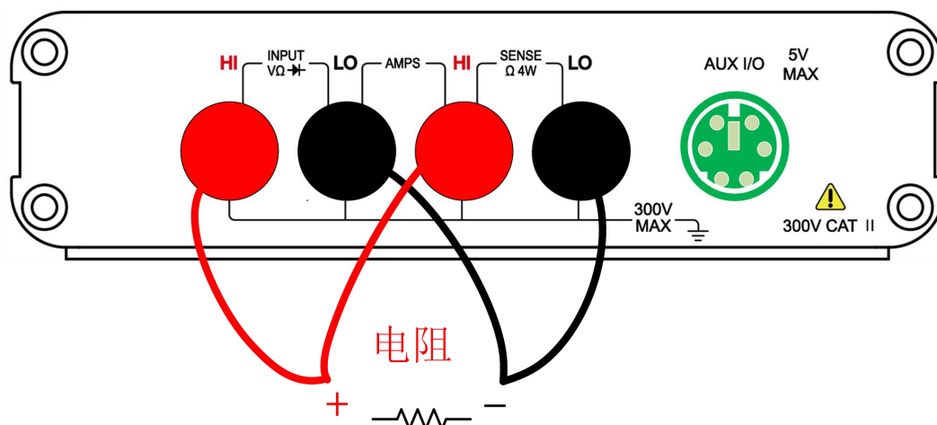
图 3-7 4W 电阻测量接线方式
