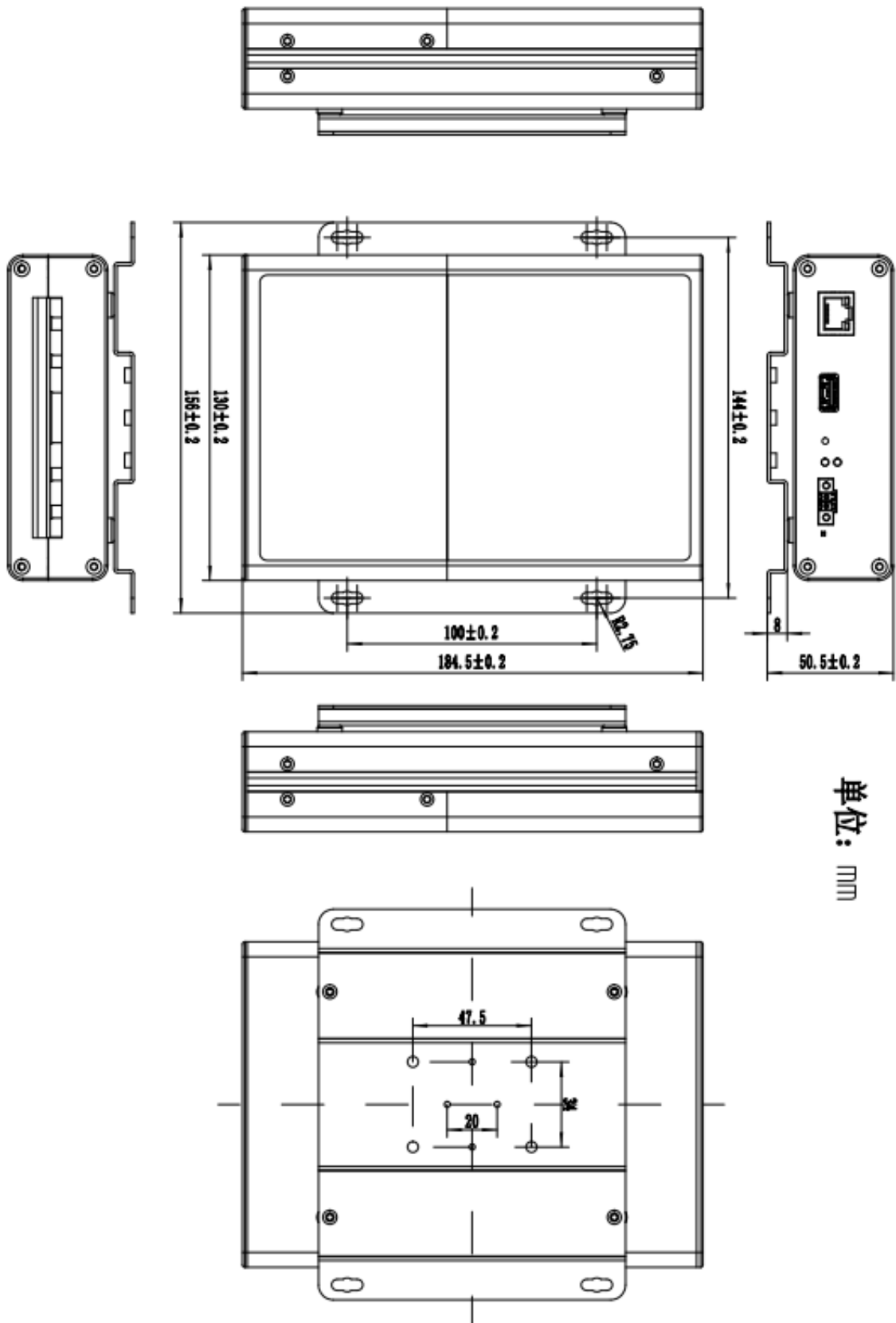
图 3-2-1 外壳尺寸图
