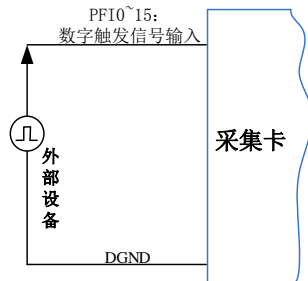
图8-3-8 数字触发连接方法
