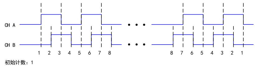
图 6-7-3 X4 编码
