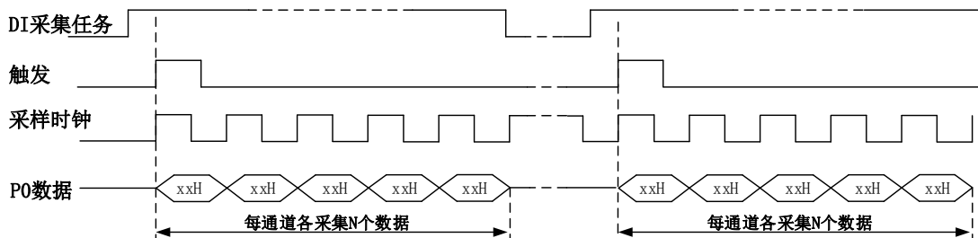
图 7-5-2 有限点采样
