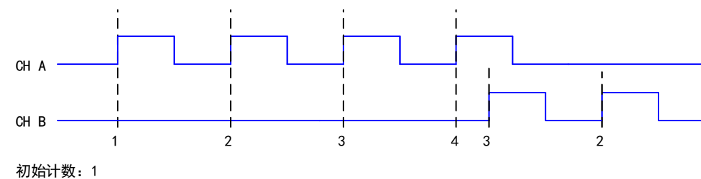
图 6-7-4 双脉冲编码
