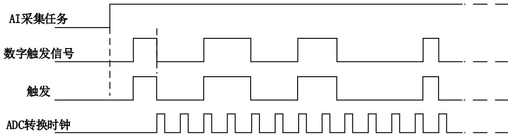
图8-2-2 数字触发--下降沿触发
