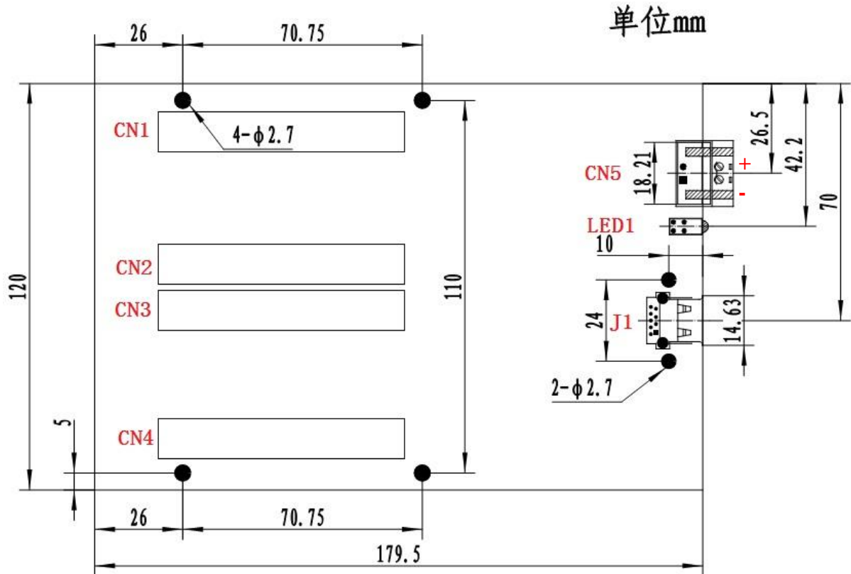
图 3-2-2 板卡尺寸图
