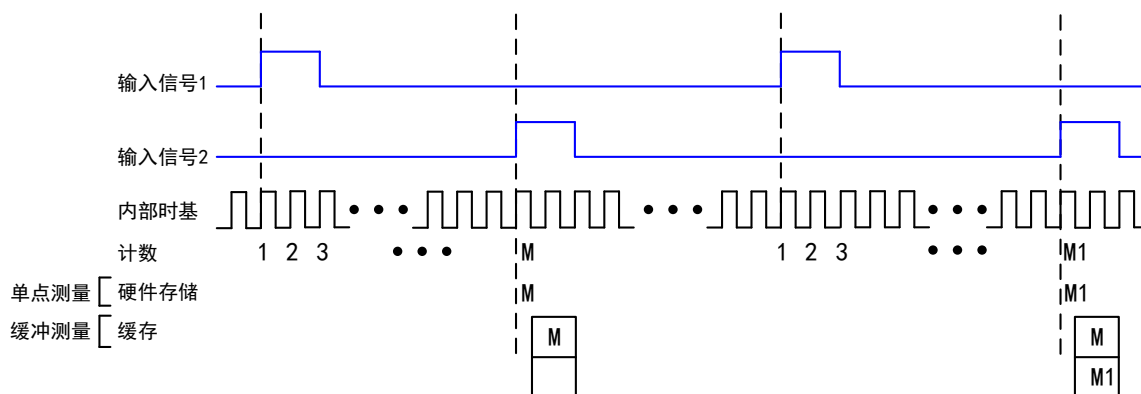
图 4-5-1 两边沿均上升沿有效示意图
