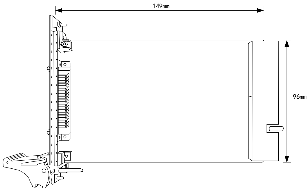
图 3-1-1 PXI2391 尺寸图
