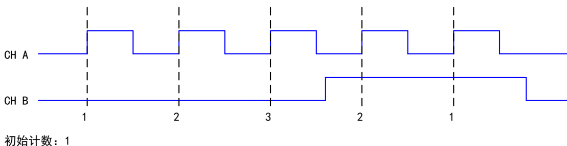
图 4-6-5 单脉冲编码
