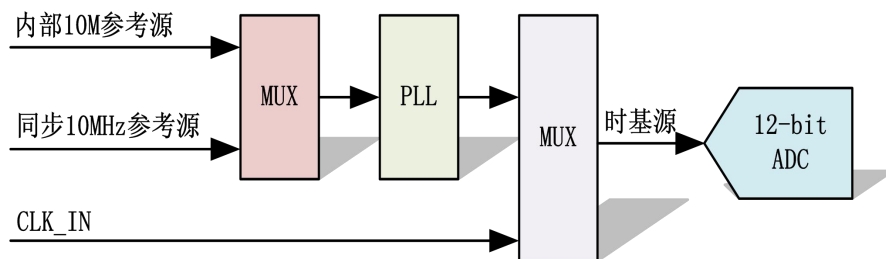
图 4-7-1 时基源框图
