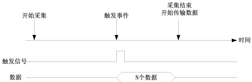
图 4-10-3 后触发
