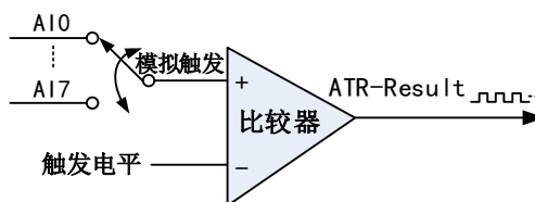
图4-8-5 比较器
