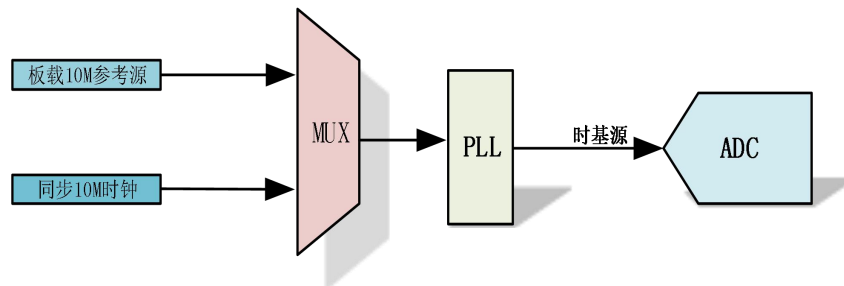
图 4-7-1 时基源框图
