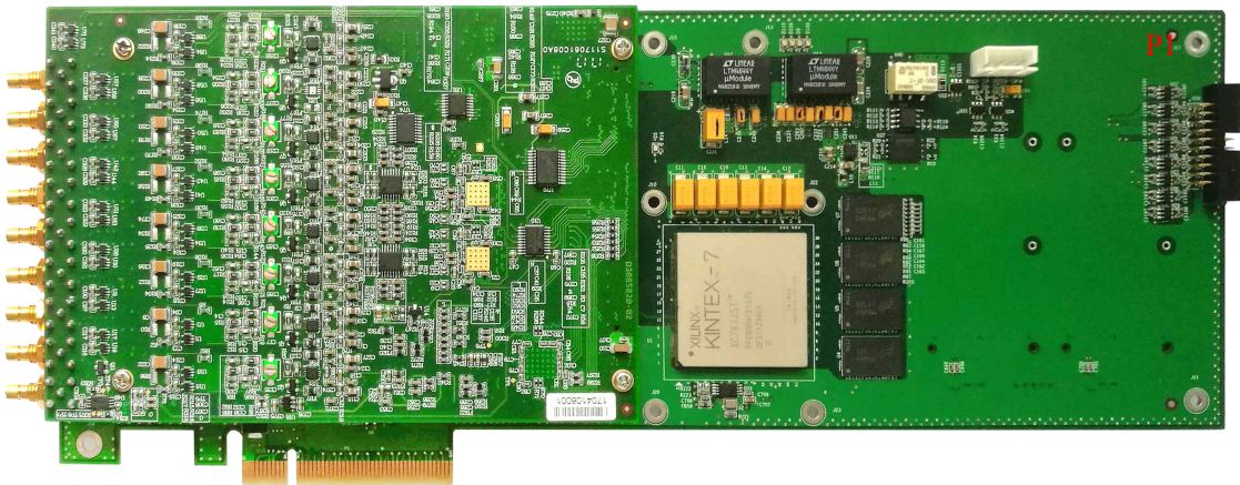
图 3-3-1 PCIe8582/8584 产品外观图
