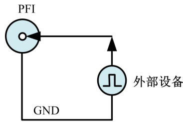
图 4-8-7 DTR 触发信号连接
