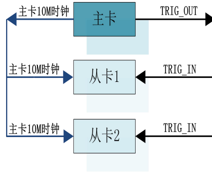
图 4-10-1 主从卡级联
