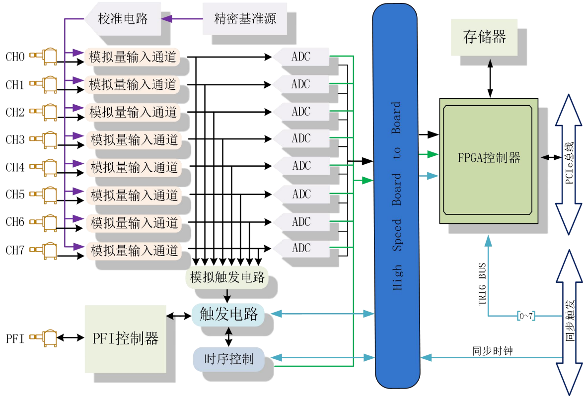
图 3-1-1 PCIe8582/8584 系统框图
