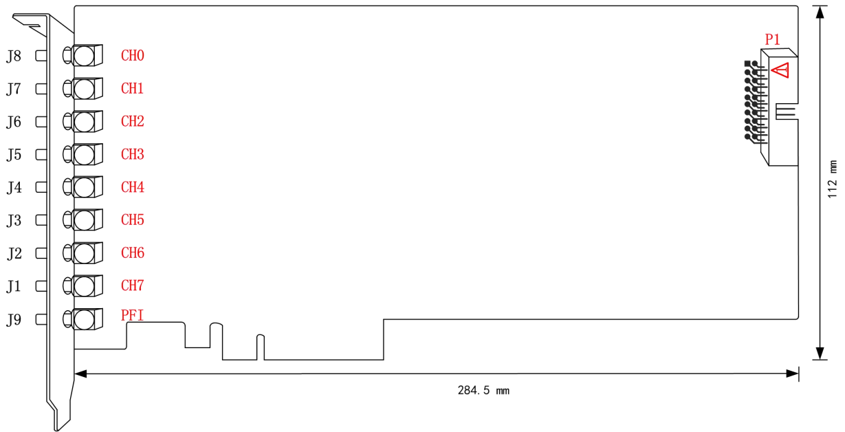
图 3-2-1 PCIe8582/8584 板卡尺寸图
