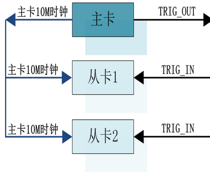
图 4-10-1 主从卡级联
