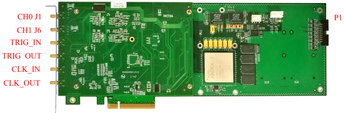
图 3-3-1 PCIe8914/8912 产品外观图
