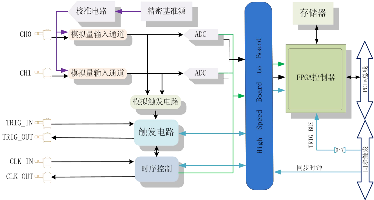
图 3-1-1 PCIe8914\8912 系统框图
