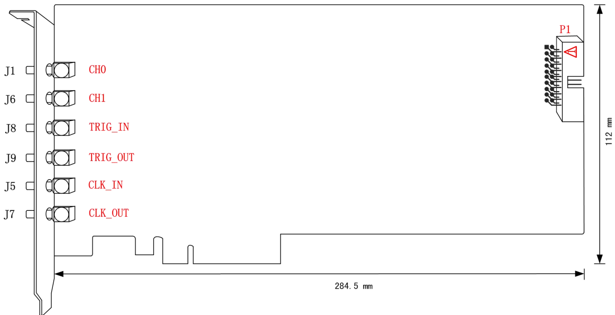
图 3-2-1 PCIe8914\8912 板卡尺寸图
