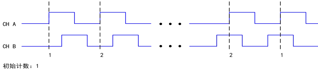
图 6-7-1 X1 编码
