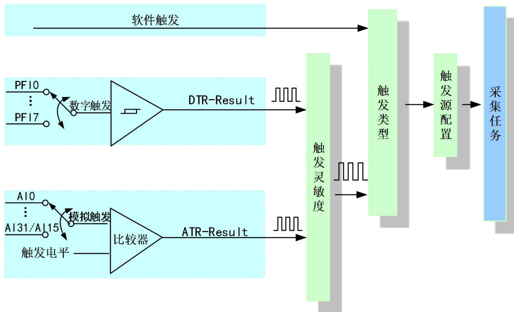
图 8-1-1 触发源选择
