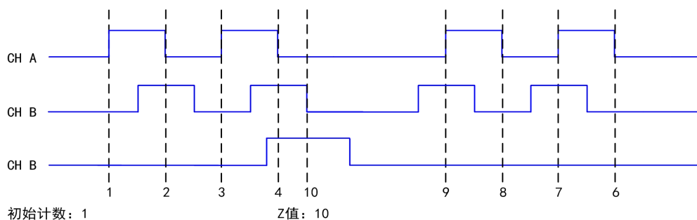
图 6-7-6 Z 索引
