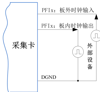
图 7-4-1 时钟输入输出的连接
