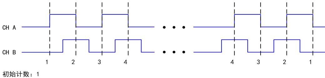
图 6-7-2 X2 编码
