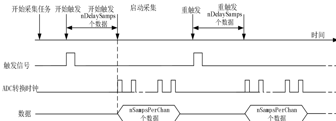
图 8-2-7 重触发
