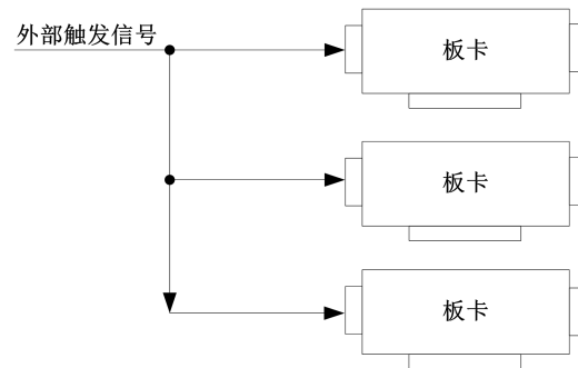
图4-10-3 外时钟同步采集的连接方式
