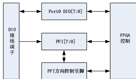
图7-1-1 DIO功能框图
