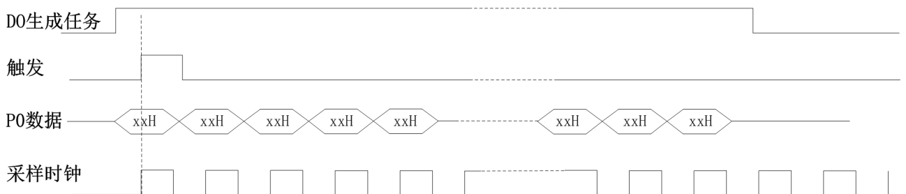
图7-6-3 内、外时钟连续生成
