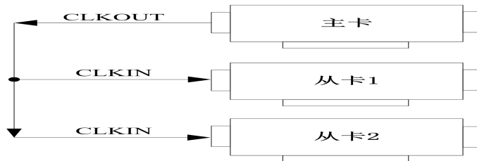
图 4-10-1 主从卡级联同步采集的连接方式
