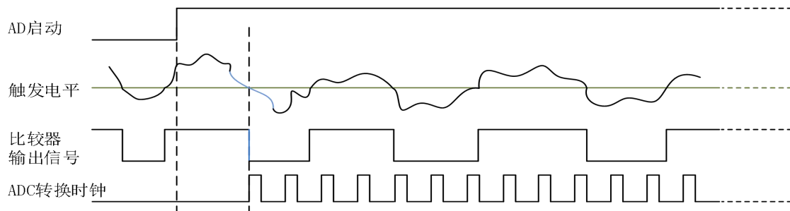
图8-2-2 模拟触发--下降沿触发
