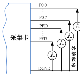
图7-2-1 DI 数字量输入的连接
