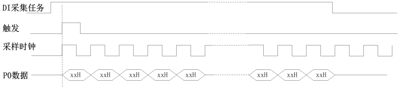
图 7-5-3 DI 连续采样
