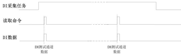
图7-5-1 按需单点采集
