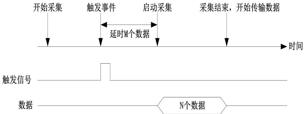
图 8-2-4 硬件延时触发
