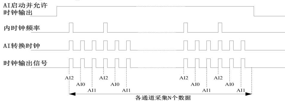
图 4-7-2 内时钟时序图
