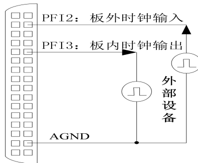
图 5-6-1 时钟输入输出的连接
