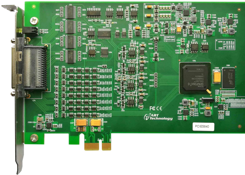
图 3-1-1 PCIe5640/1/2/3 正面图
