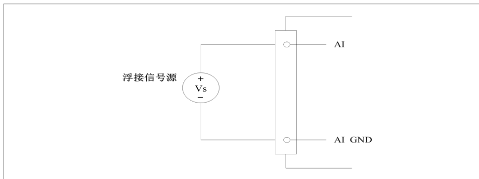
图 4-5-5 浮接信号源的参考地单端 (RSE) 连接
