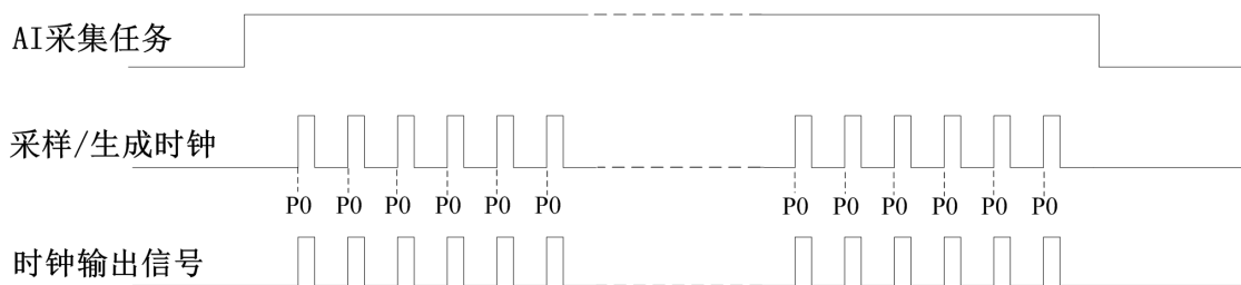
图 7-4-3 外时钟时序图
