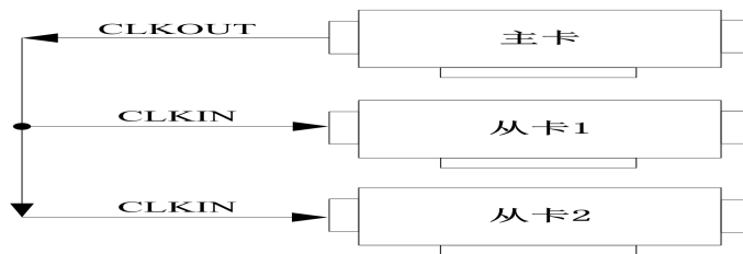
图 4-10-2 主从卡级联同步采集的连接方式
