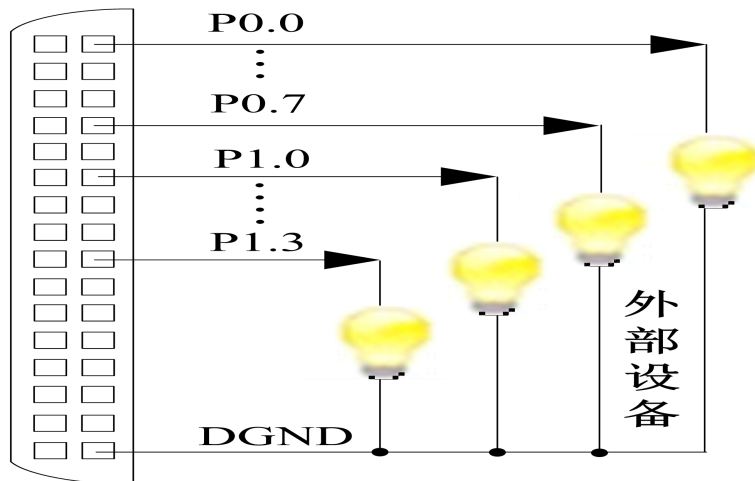
图 7-3-3 DO 数字量控制继电器电路
