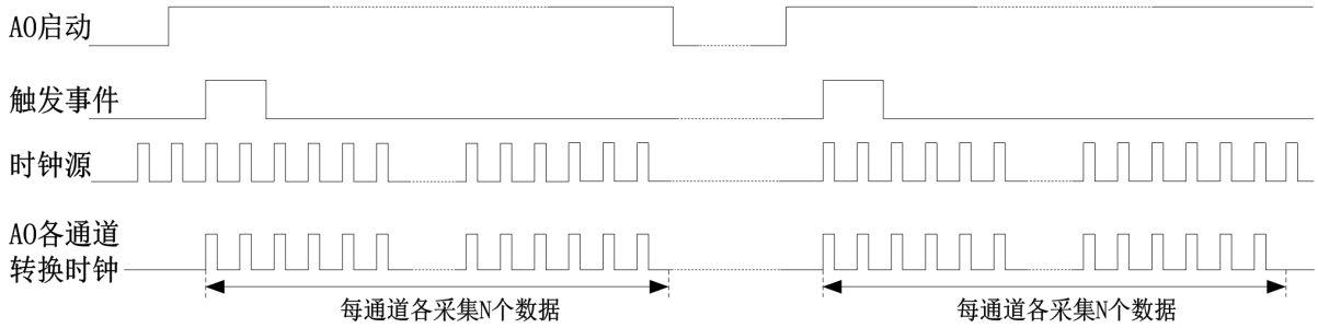
图5-7-2 内、外时钟有限点生成
