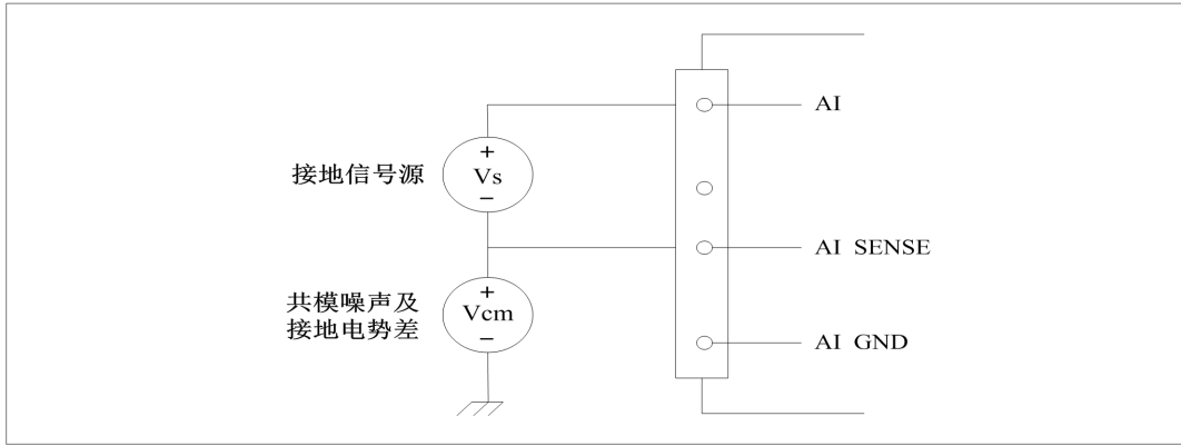
图 4-5-7 接地信号源的无参考地单端（NRSE）连接
