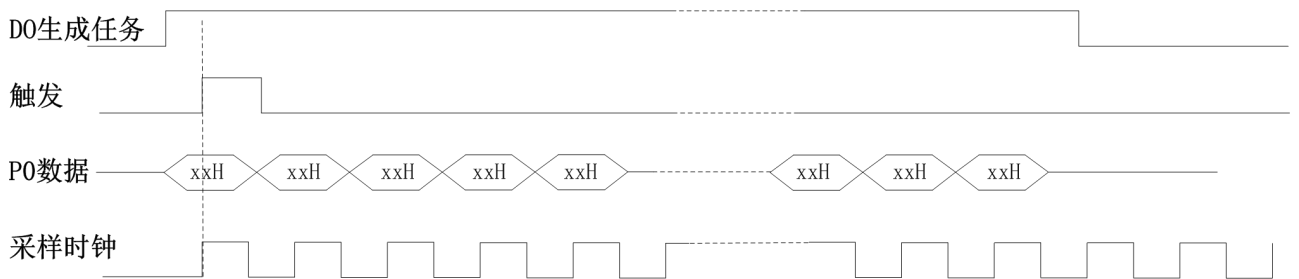
图7-6-3 内、外时钟连续生成
