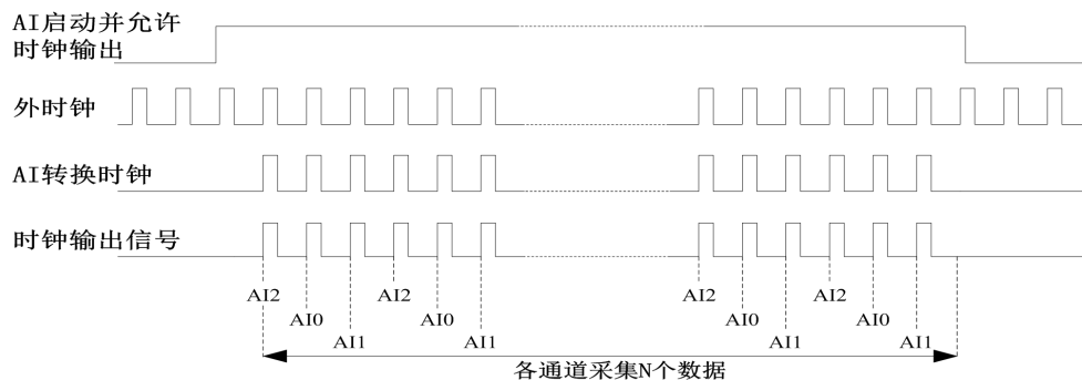
图 4-7-3 外时钟时序图
