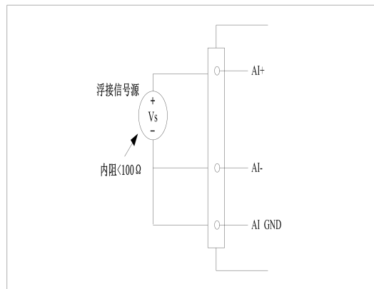
图 4-5-1 浮接信号源差分（DIFF）连接 -- 直接连接
