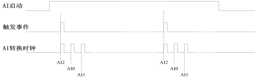
图4-8-1 按需单点采集
