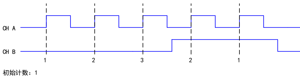
图 6-6-5 单脉冲编码
