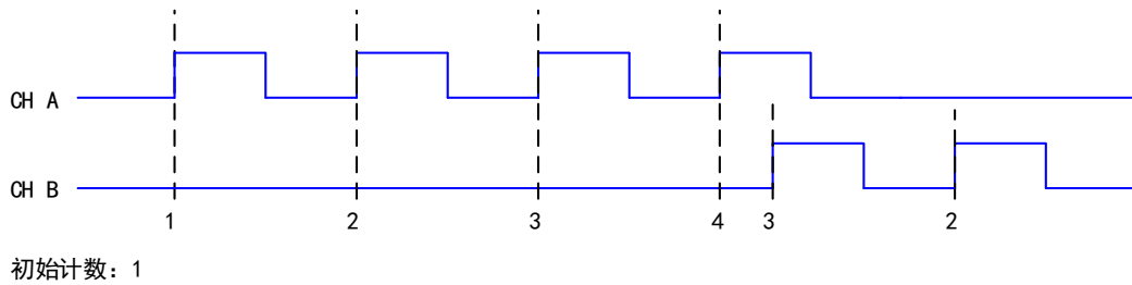
图 6-6-4 双脉冲编码
