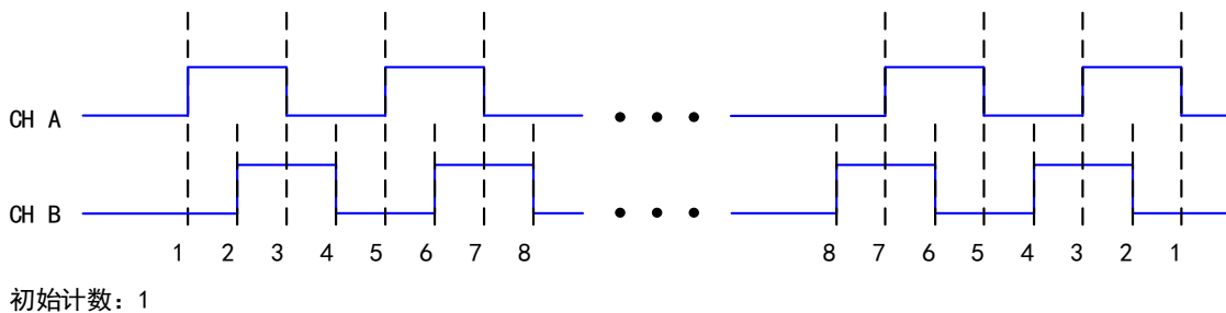
图 6-6-3 X4 编码
