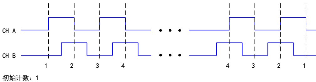
图 6-6-2 X2 编码
