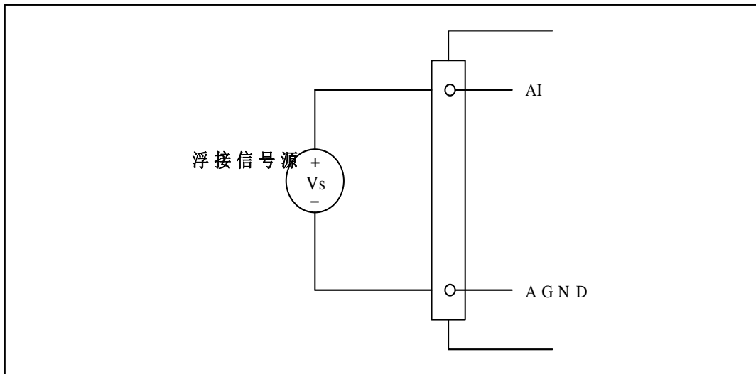
图 4-4-5 浮接信号源的参考地单端（RSE）连接
