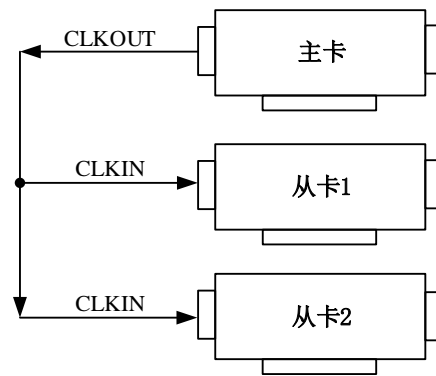
图 4-10-1 主从卡级联
