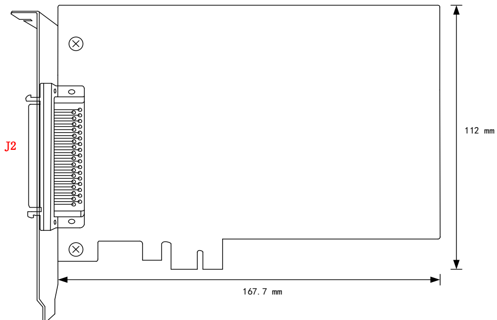
图 3-2-1 尺寸图
