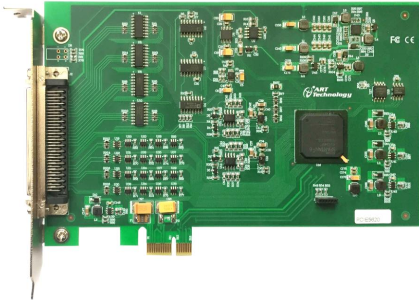
图 3-1-1 PCIe5620 正面图
