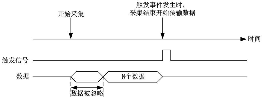
图 4-10-4 预触发
