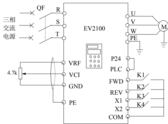
图5-55 两地控制硬件接线图
