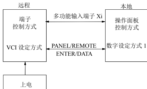
图5-54 两地控制需求
