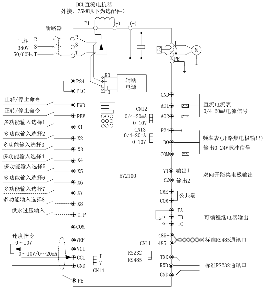
图3-10 基本配线图2
