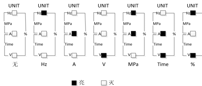
图4-3 单位指示灯状态与单位对应关系图
