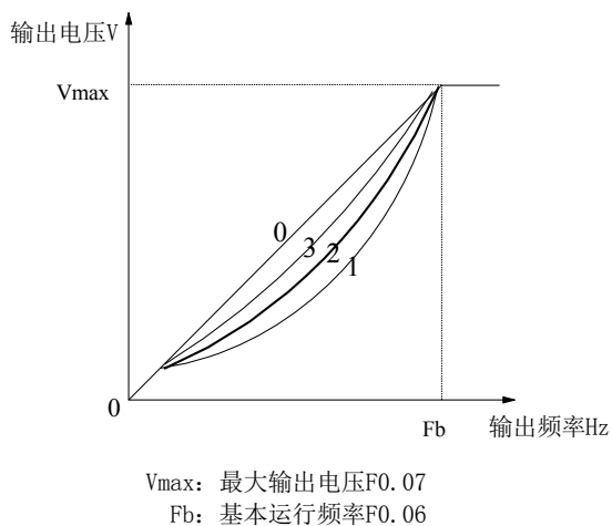
图5-5 降转矩曲线
