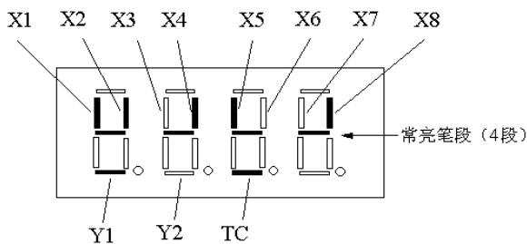
图5-52 端子状态指示
