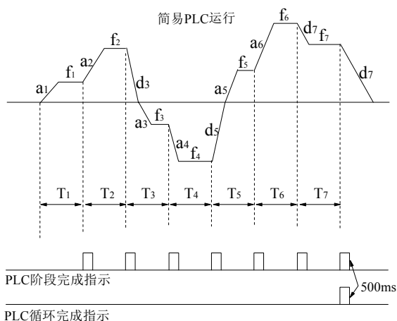
图5-16 简易PLC运行图
