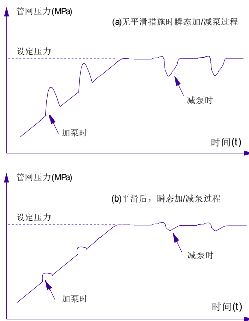
图5-36 有无平滑措施时加/减泵过程对比示意图
