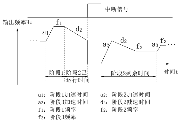
图5-22 PLC起动方式2
