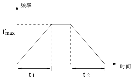
图5-12 直线加减速
