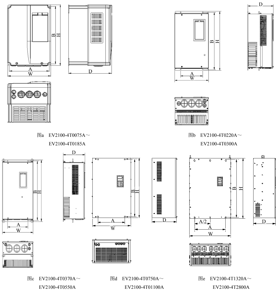
图2-2 变频器外形尺寸图
