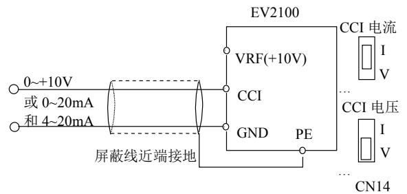
图3-14 CCI端子配线图
