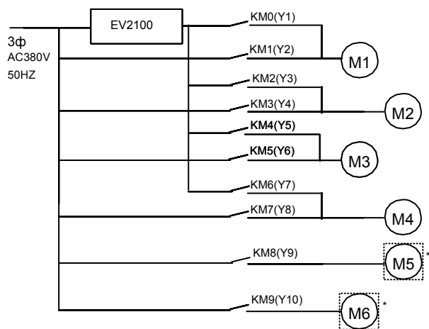
图5-34 F6.01=3或8 (4泵变频循环方式) 最大配置示意
