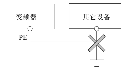
图3-38 接地示意图3
