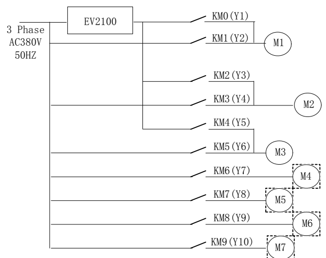
图5-33 F6.01=2或7 (3泵变频循环方式) 最大配置示意图
