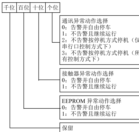
图5-64 保护动作选择1设定
