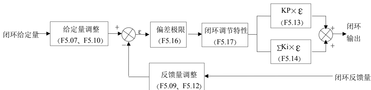
图5-25 PI原理框图
