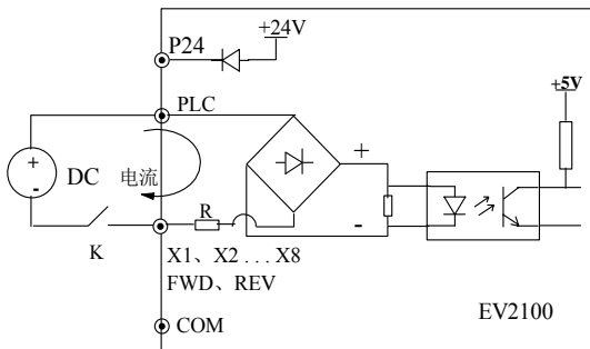
图3-22 使用外部电源的连线方式
