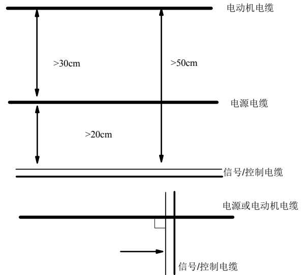
图3-33 系统配线要求
