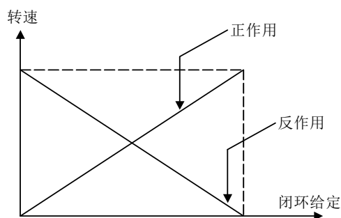
图5-27 闭环调节特性示意图
