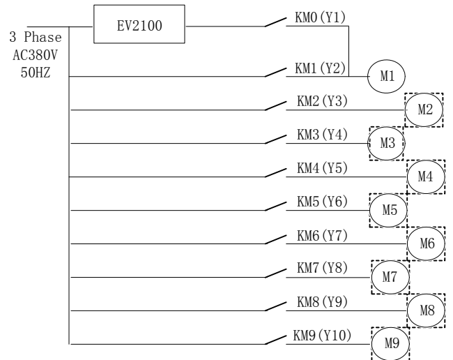
图 5-31 F6.01=0 或 5 (变频固定方式) 最大配置示意图
