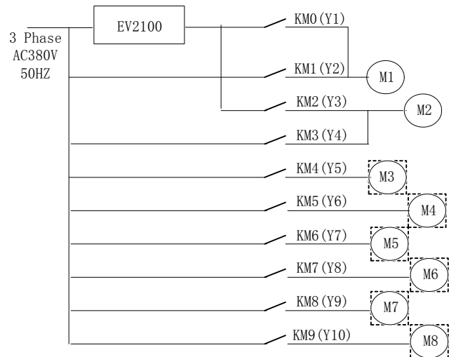
图5-32 F6.01=1或6 (2泵变频循环方式) 最大配置示意图
