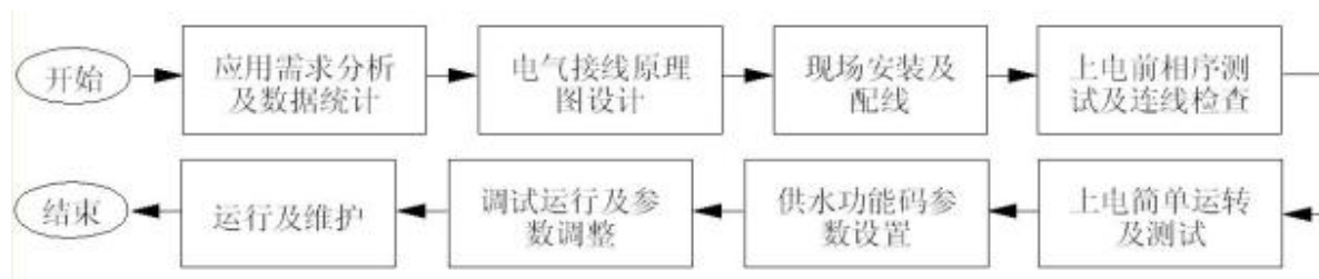
附图15 供水应用基本步骤框图
