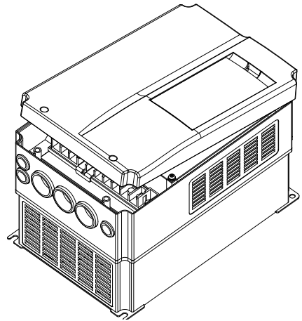
图3-5 塑胶盖板的拆卸和安装示意图
