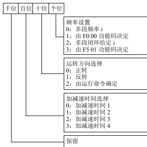
图5-23 PLC阶段i设置 (i=1~7)
