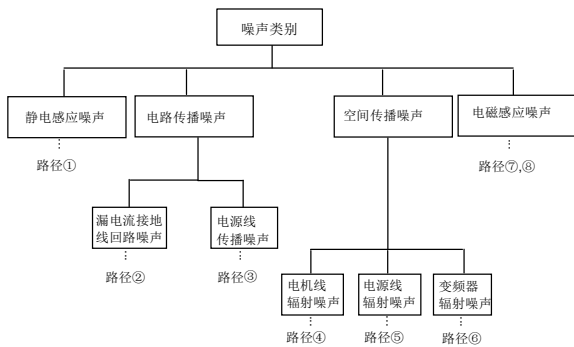
图3-31 噪声分类
