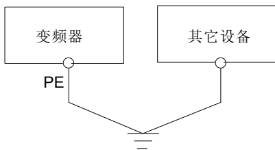
图3-37 接地示意图2
