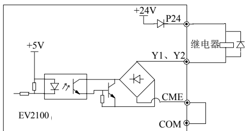
图3-27 多功能输出端子接线方式1
