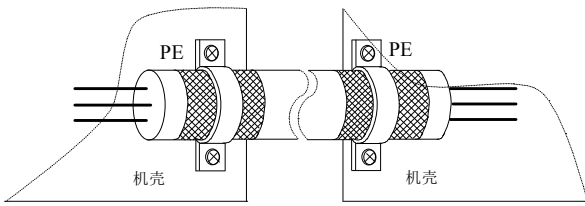
图3-34 正确的屏蔽接地方法
