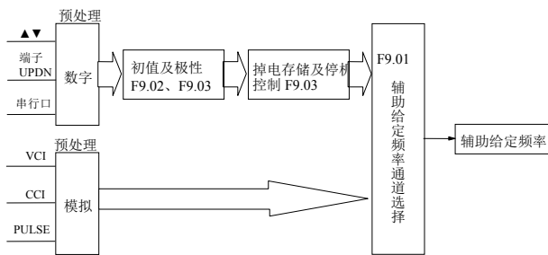
图5-57 辅助频率给定通道示意图
