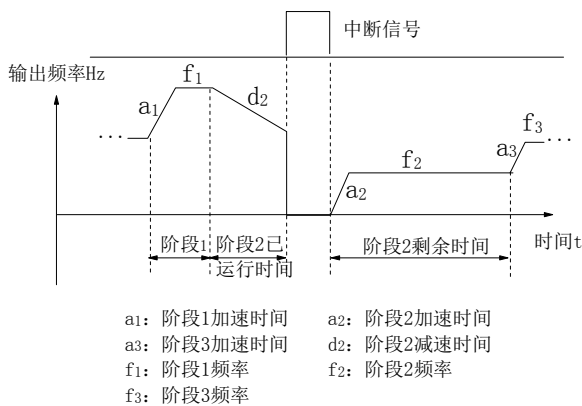
图5-21 PLC启动方式1
