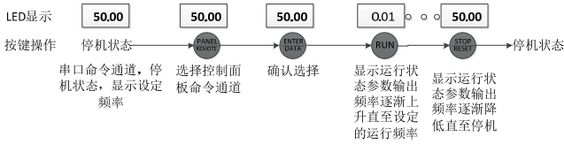
图4-10 运行与停机的操作示例
