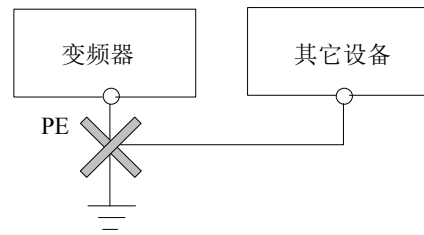
图3-39 接地示意图4
