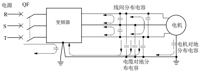
图3-41 漏电流路径
