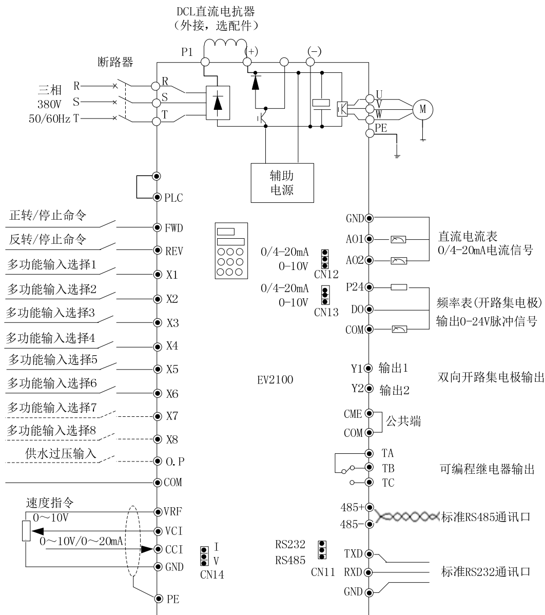
图3-9 基本配线图1
