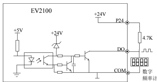
图3-29 输出端子DO连接方式1
