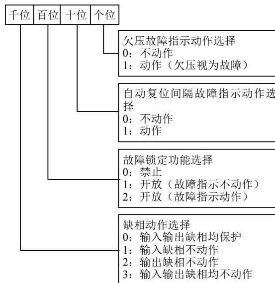
图5-65 保护动作选择2设定
