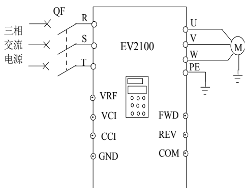
图3-7 主回路简单配线图
