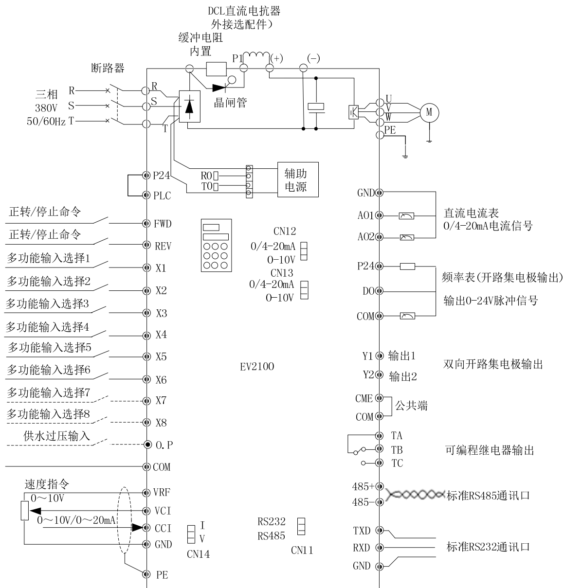
图3-11 基本配线图3
