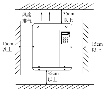
图3-2 安装的间隔距离 (75kW及以上)
