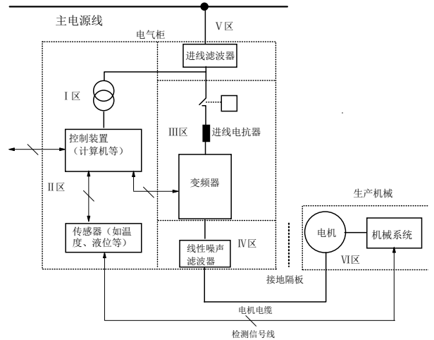
图3-42 变频器EMC安装推荐区域划分示意图
