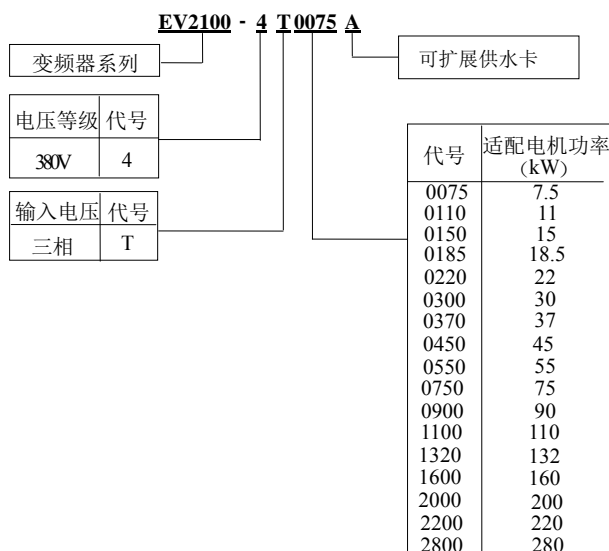
图A-1 变频器型号说明
