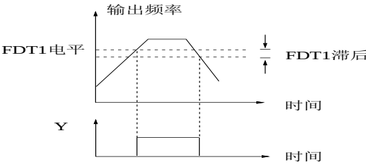
图 5-43 频率水平检测示意图
