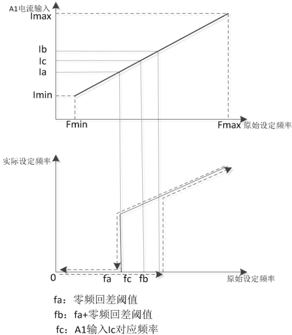
图 5-51 零频回差运行
