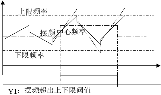
图 5-37 摆频幅度限制
