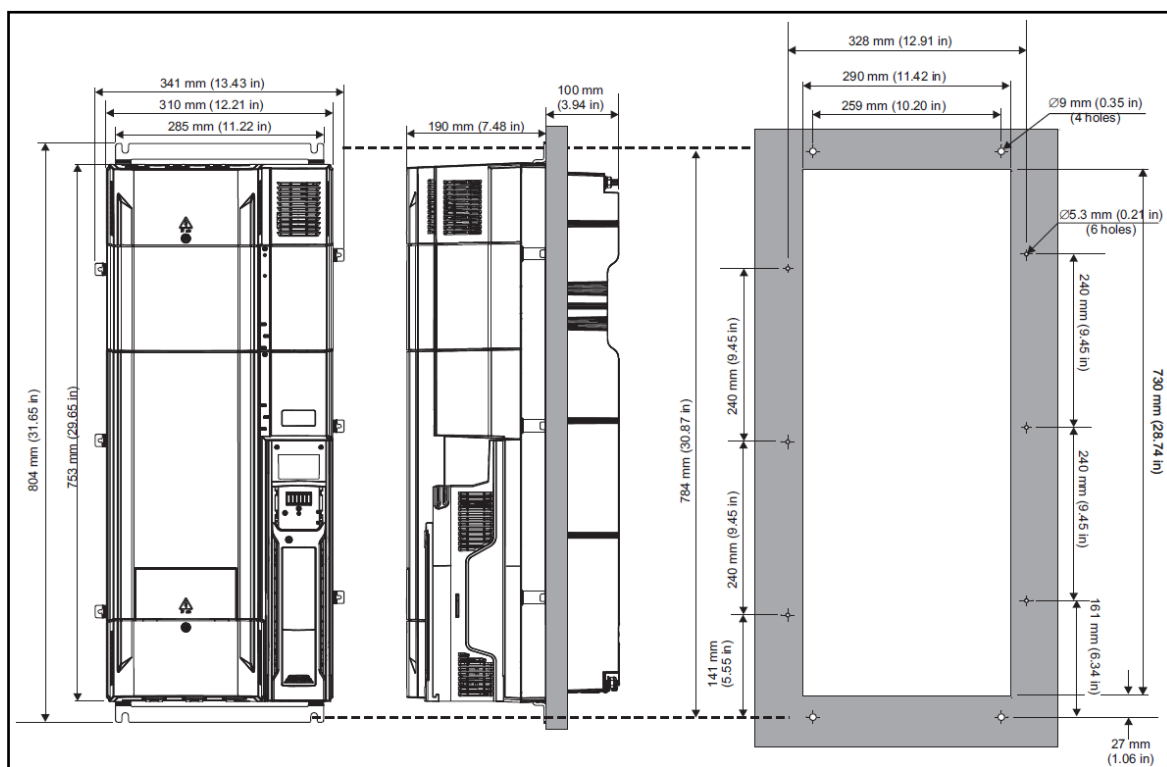
图 3-14 Size8 透壁式安装尺寸图
