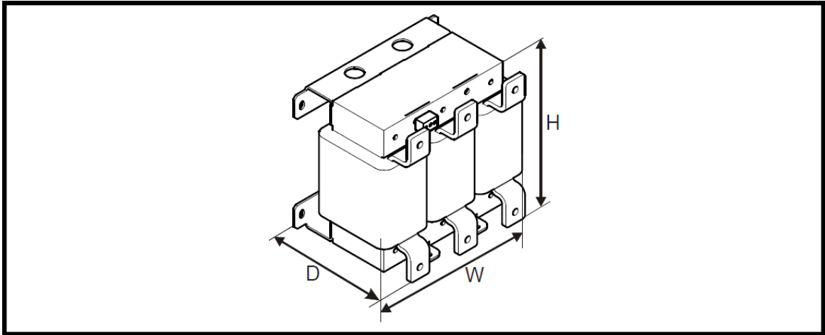
附图 3 交流输入电抗器外形图（4402-0227，4402-0228，4402-0229）
