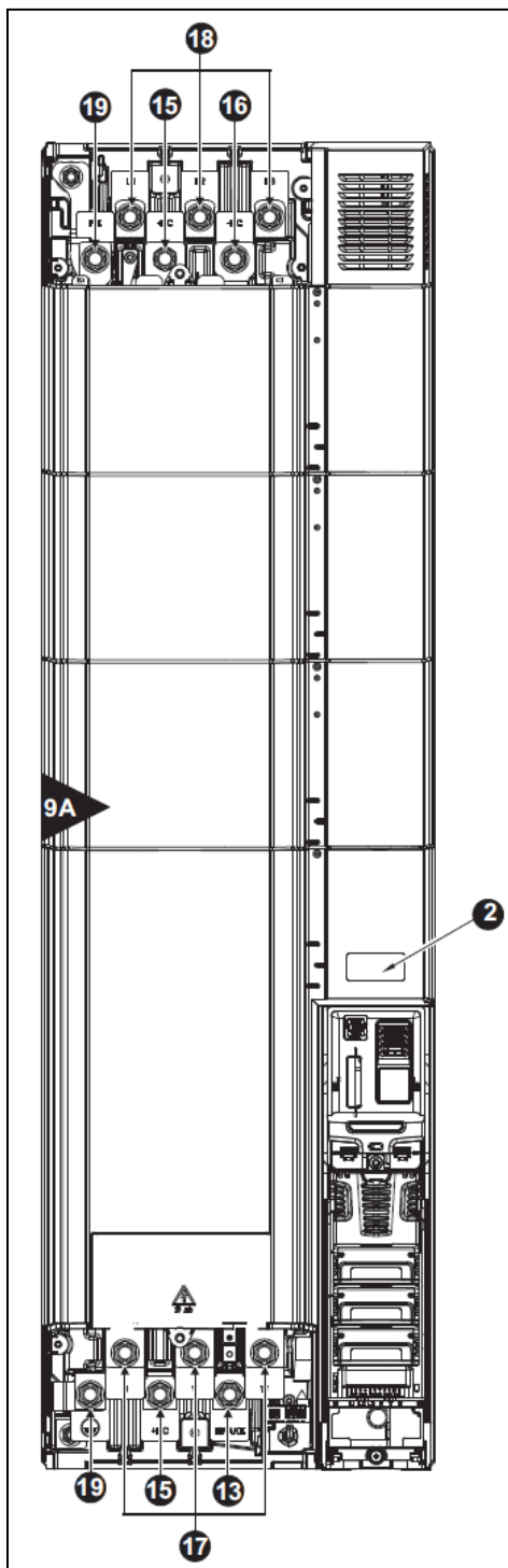
图 2-3 Size 9A (90k - 110kW)变频器各部位名称示意图
