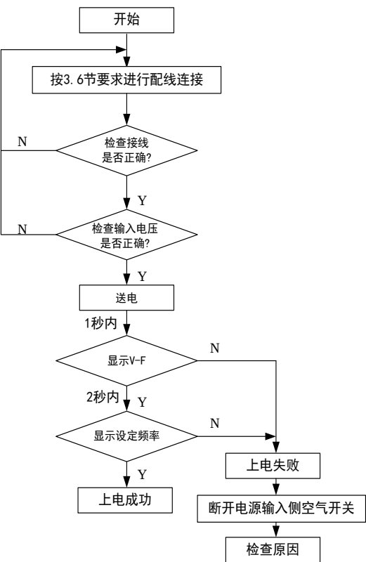
图 4-11 变频器初次上电操作流程
