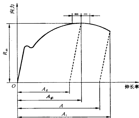
图1 伸长的定义
