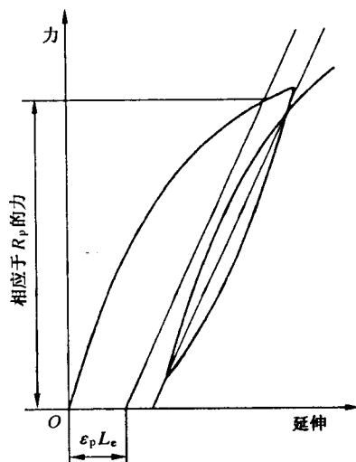
图 7 规定非比例延伸强度( R_p )(见 15.1)
