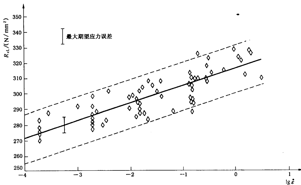
图 J1 板钢的下屈服强度 R_{eL} 随应变速率的变化(室温)
