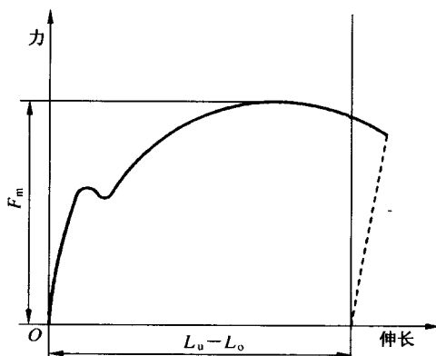
图 8 最大力( F_m )
