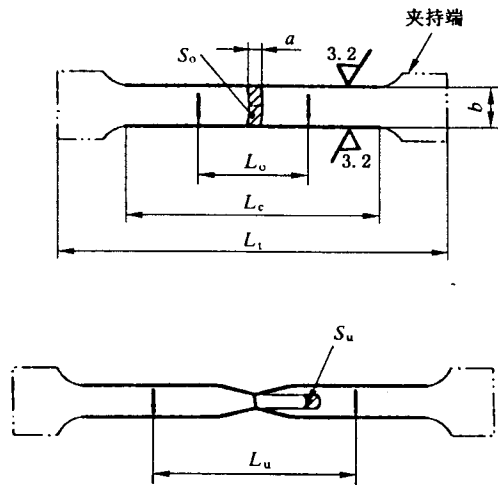
图 13 管的纵向弧形试样(见附录 D)
