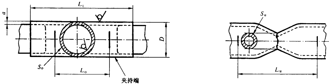
图 13 管的纵向弧形试样(见附录 D)
