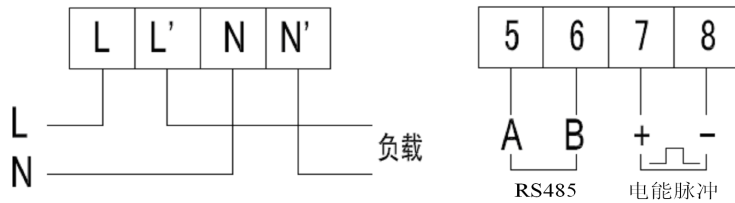
DDSY1352-NK 接线图
