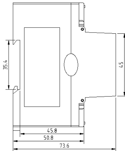
左视
