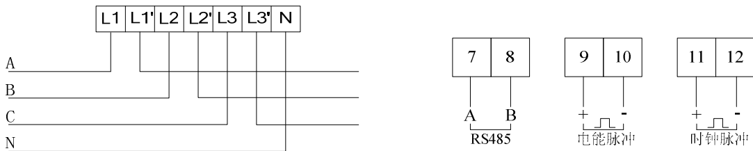
DTSY1352-NK 接线图
