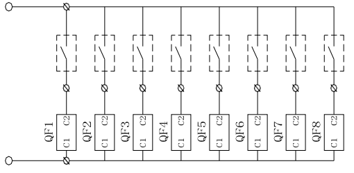
分 例 脱 扣 器 回 路
