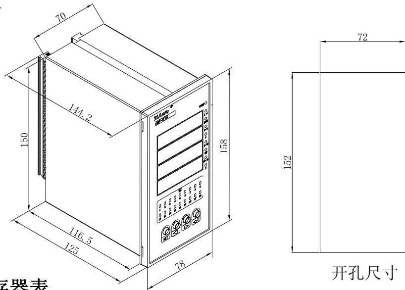
16 外形安装尺寸
