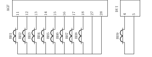
电 流 测 量 回 路
