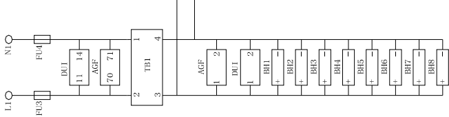
电 压 测 量 及 供 电 回 路
