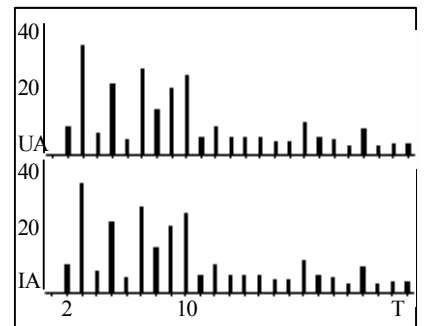
谐波棒图
