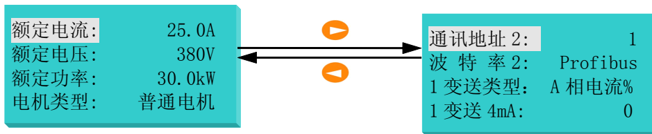
图 35 profibus 从站设定
