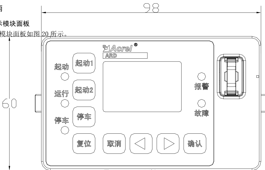
图 20 60L 显示面板
