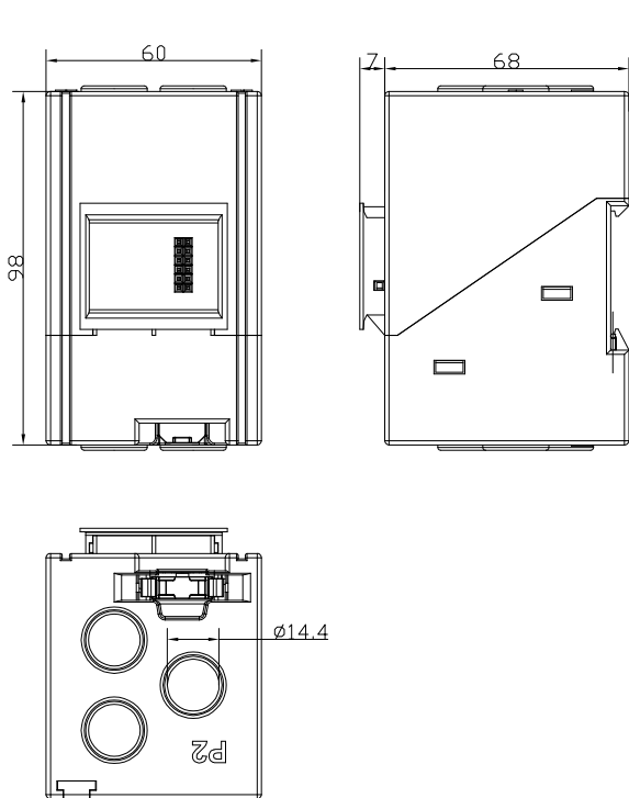
图5 电流测量模块尺寸
