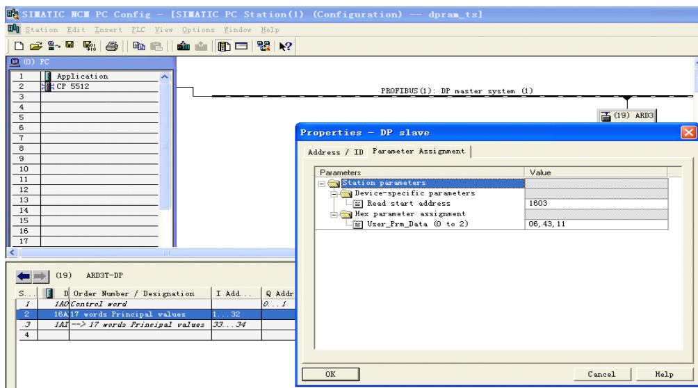
图 37 17words 输入数据用户参数
