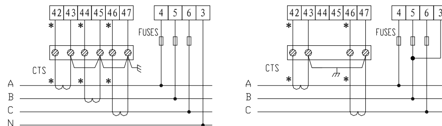
三相四线
