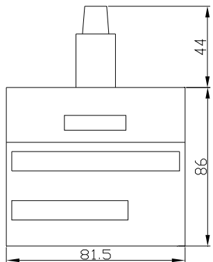
图 3 (a) ACM3 主体主视图
