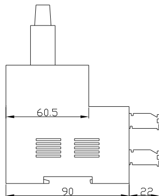
图 3 (b) ACM3 主体左视图
