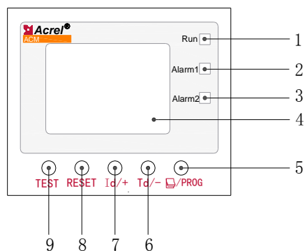
图 6 ACM2 操作面板
