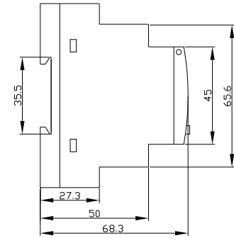
图 1 (b) ACM2 左视图
