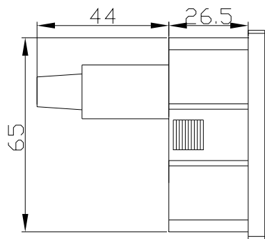
图 4 (b) 90L 显示单元左视图
