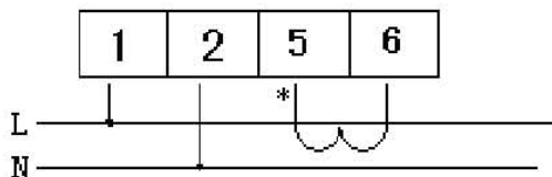
图8 接线方式
