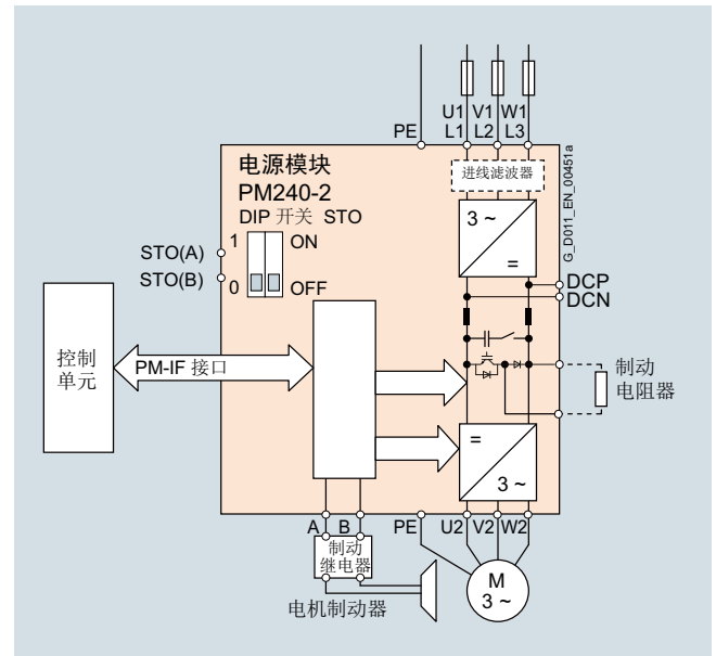
带 / 不带集成式进线滤波器、机座号为 FSD 至 FSF 的 PM240-2 电源模块的连接图
