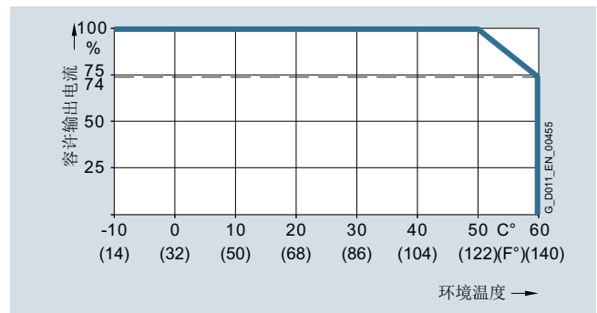
高过载 (HO) 时, 机座号为 FSA 至 FSC 的 PM240-2 电源模块的容许输出电流随环境温度的变化而变化
