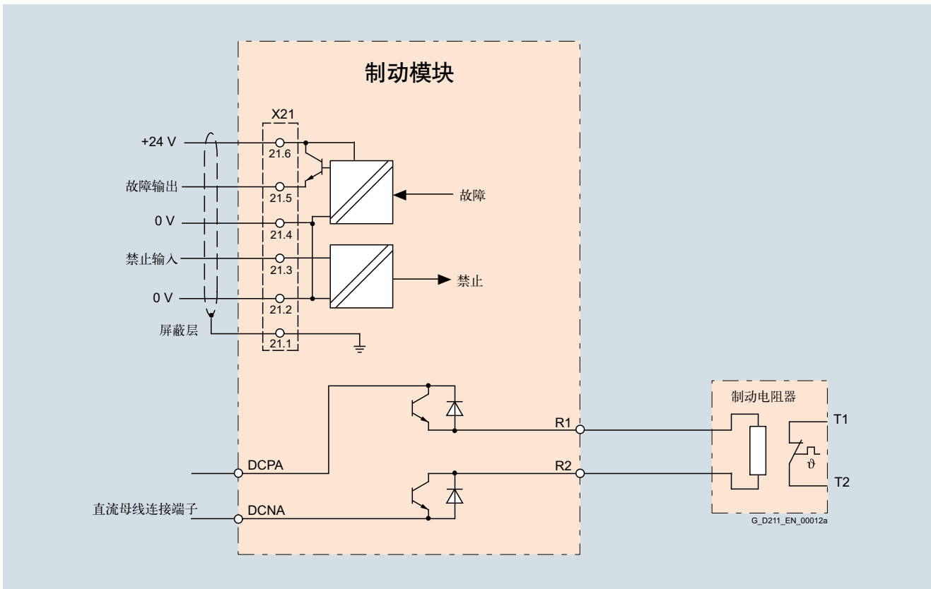
制动模块连接示例
