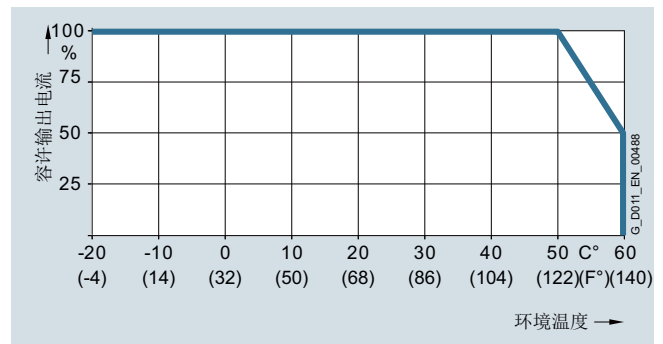
高过载 (HO) 时, 机座号为 FSD 至 FSF 的 PM240-2 电源模块的容许输出电流随环境温度的变化而变化
