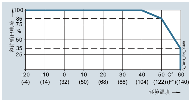
低过载 (LO) 时, 机座号为 FSD 至 FSF 的 PM240-2 电源模块的容许输出电流随环境温度的变化而变化
