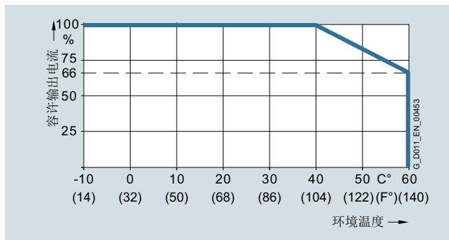
低过载 (LO) 时, 机座号为 FSA 至 FSC 的 PM240-2 电源模块的容许输出电流随环境温度的变化而变化
