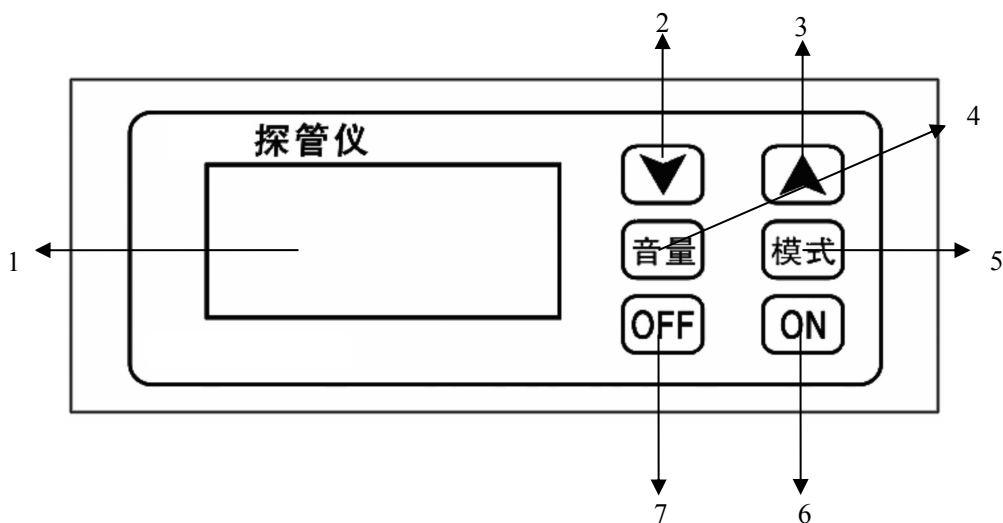
图 2 探管仪面板示意图
