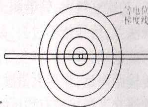
图 12 地表等电位梯度平面分布图
