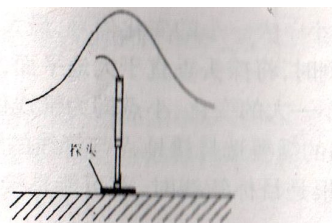
图 9 峰值法探测示意图
