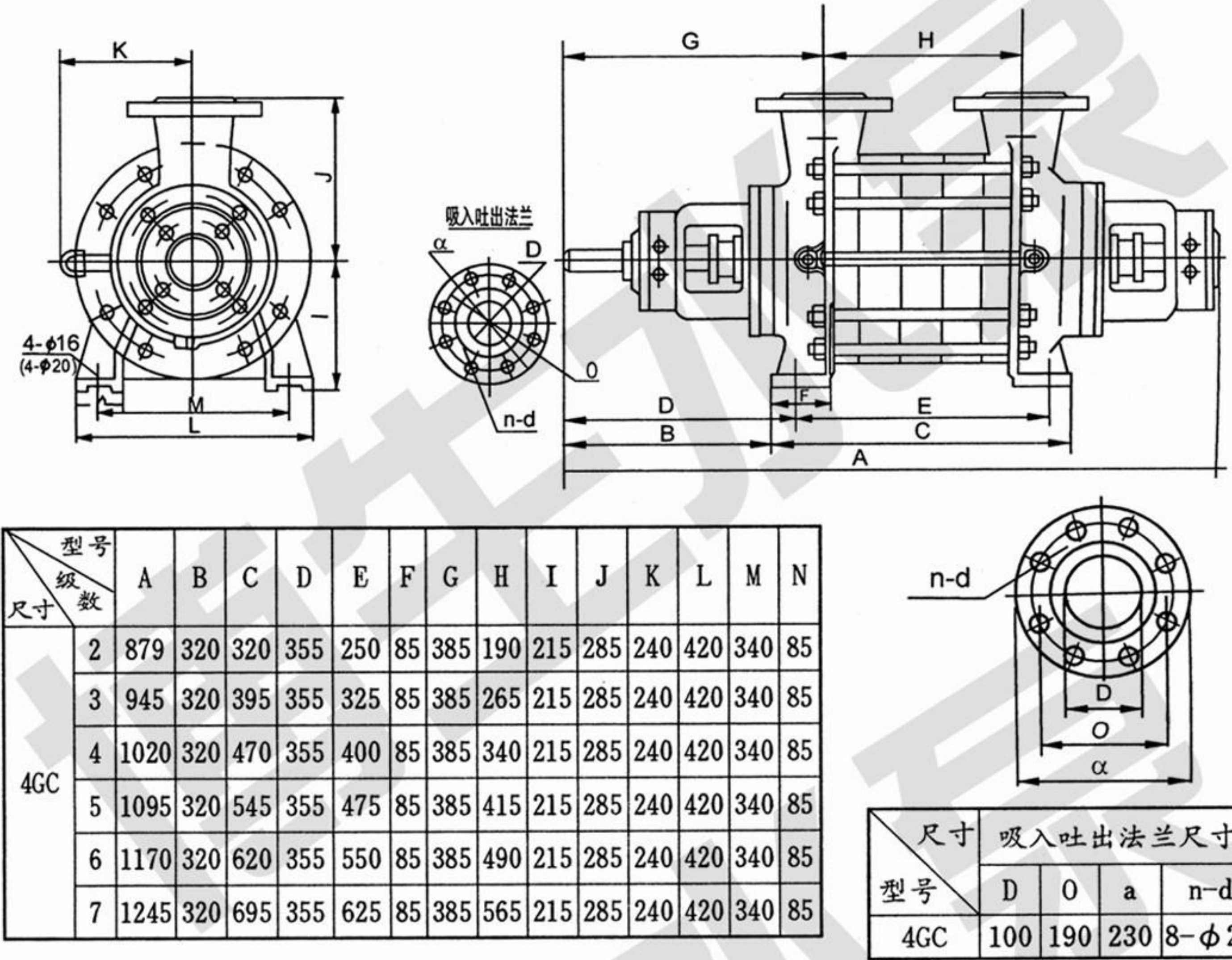
十、GC型泵安装尺寸图表与尺寸图
