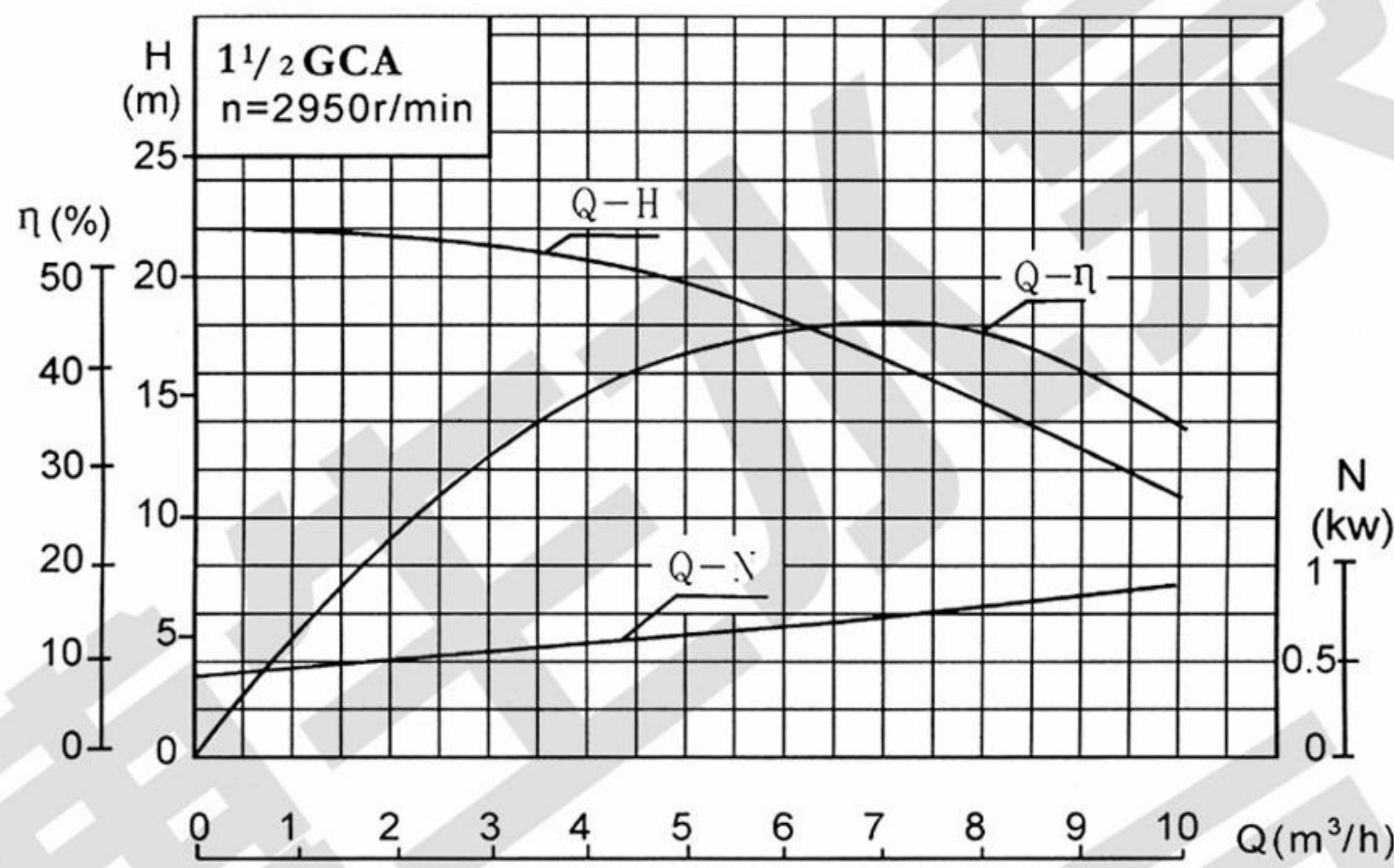
1 1/2 GCA型离心水泵性能表
