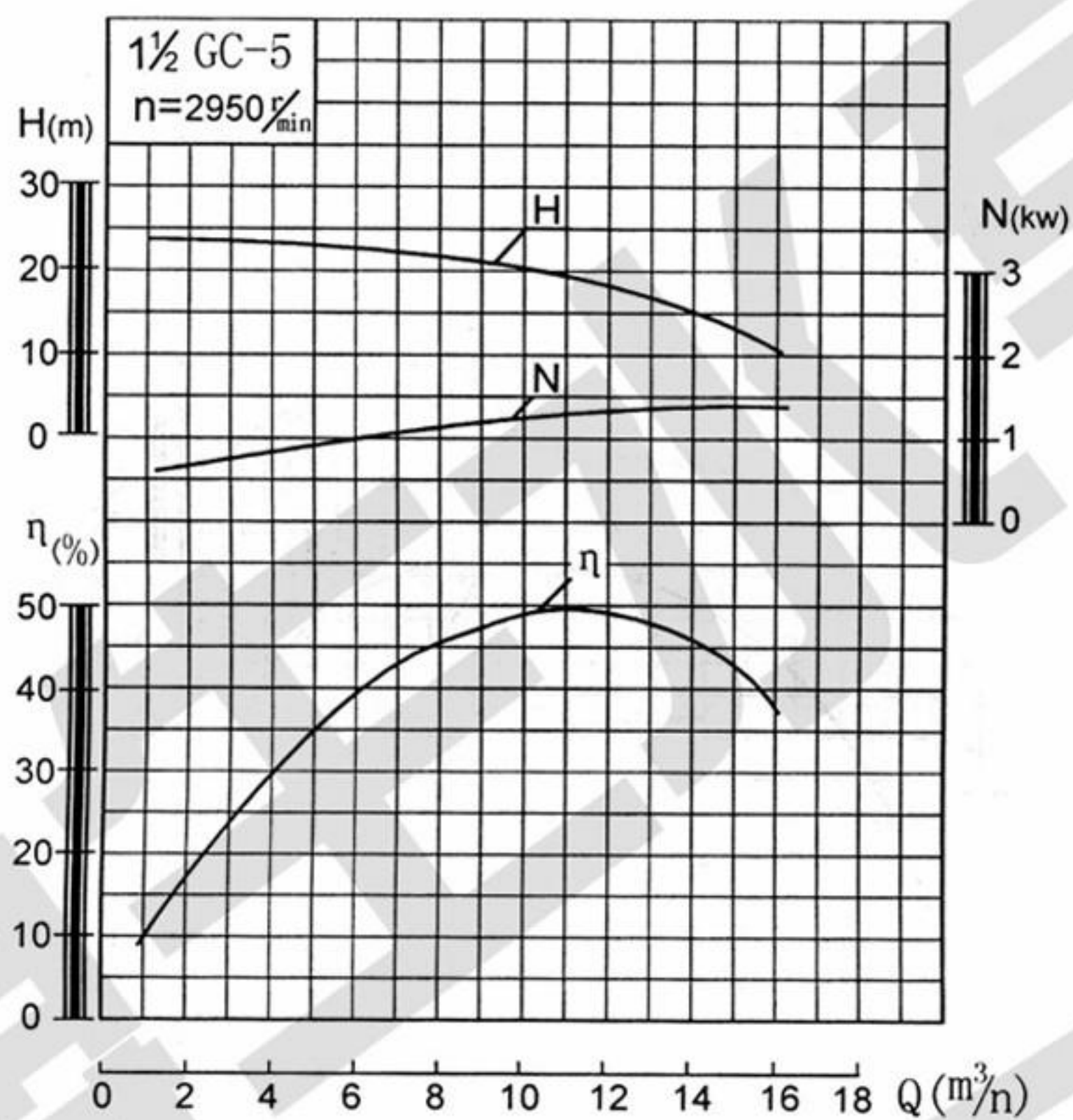
1 1/2 GC型离心水泵性能表
