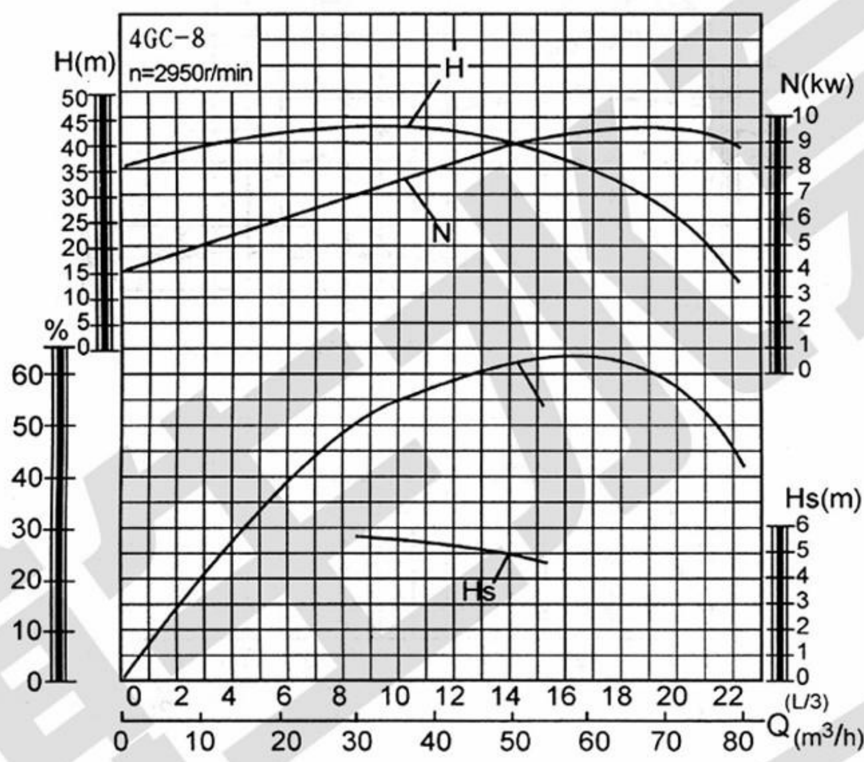
4GC型离心水泵性能表
