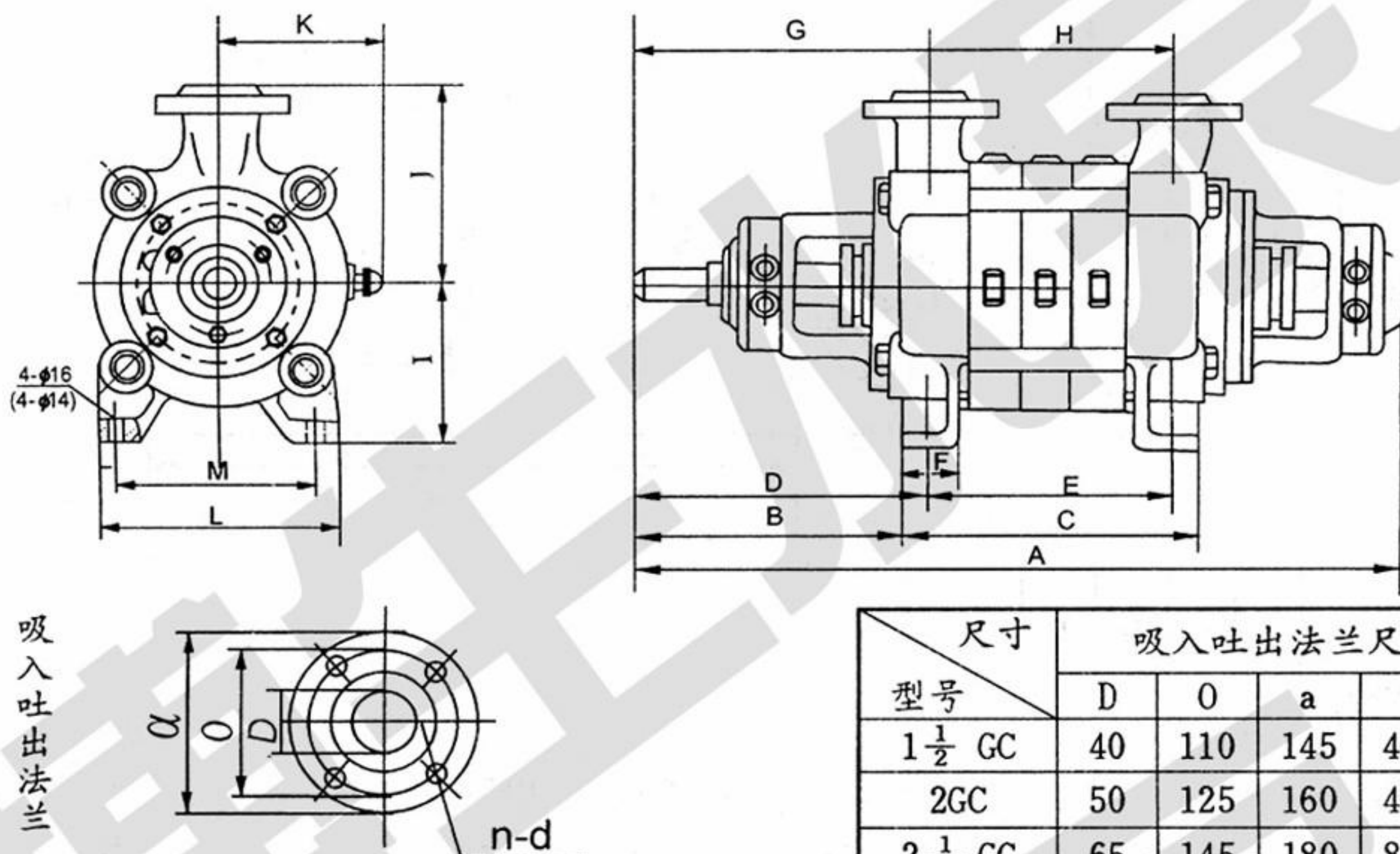
1\frac{1}{2} GC、2GC、 2\frac{1}{2} GC型离心水泵外形尺寸图
