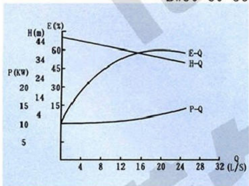
ZW80-80-35
