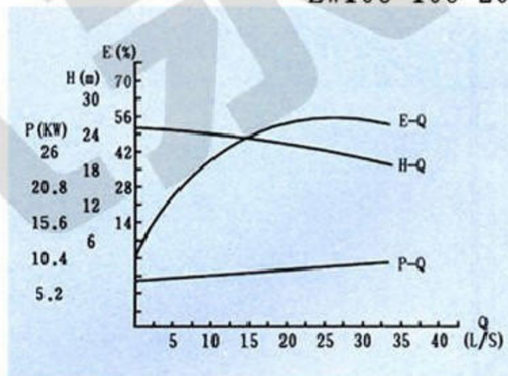
ZW100-100-20
