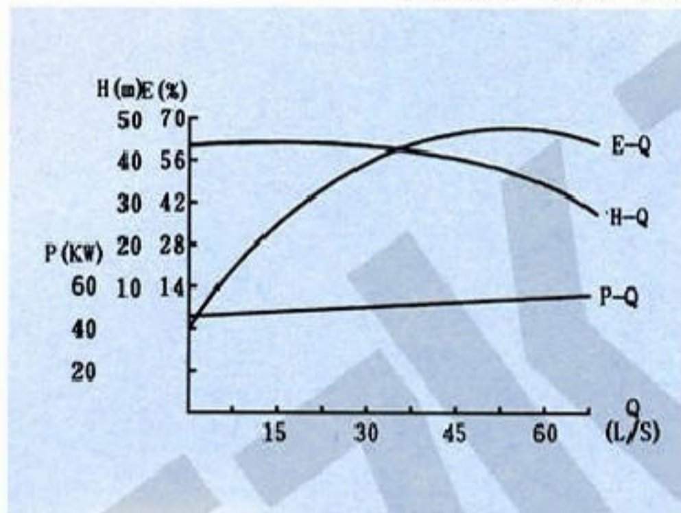
ZW150-180-38
