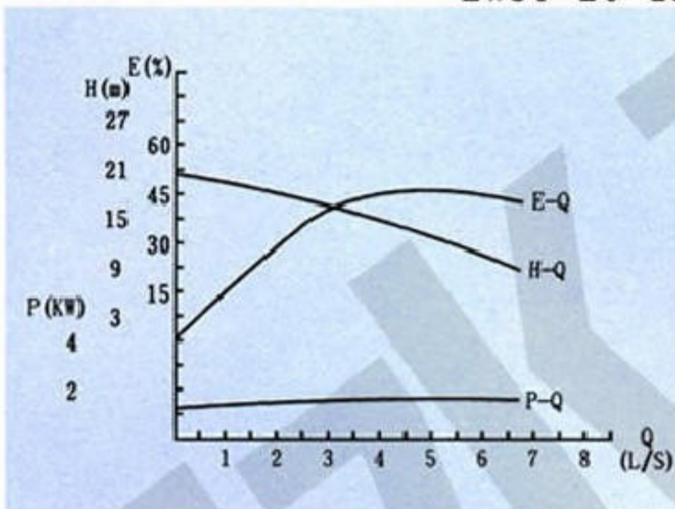
ZW50-20-12
