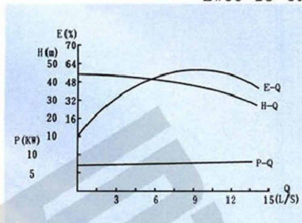
ZW65-25-40
