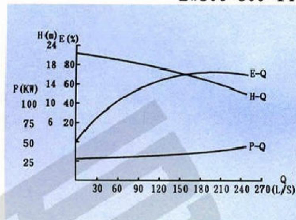
ZW300-800-14
