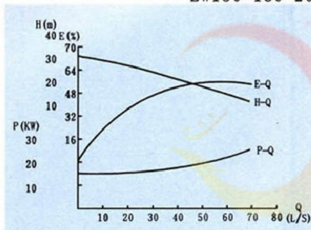
ZW150-180-20
