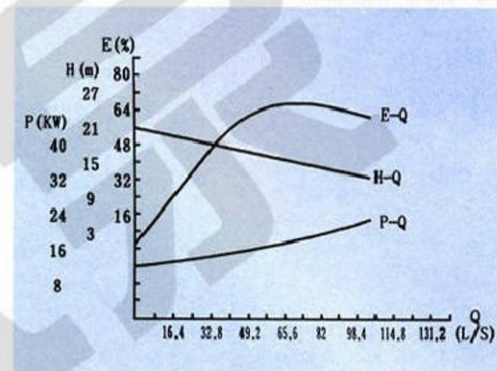
ZW200-280-14
