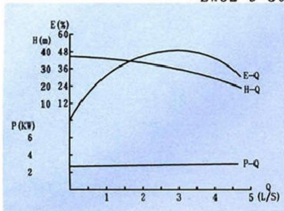
ZW32-9-30
