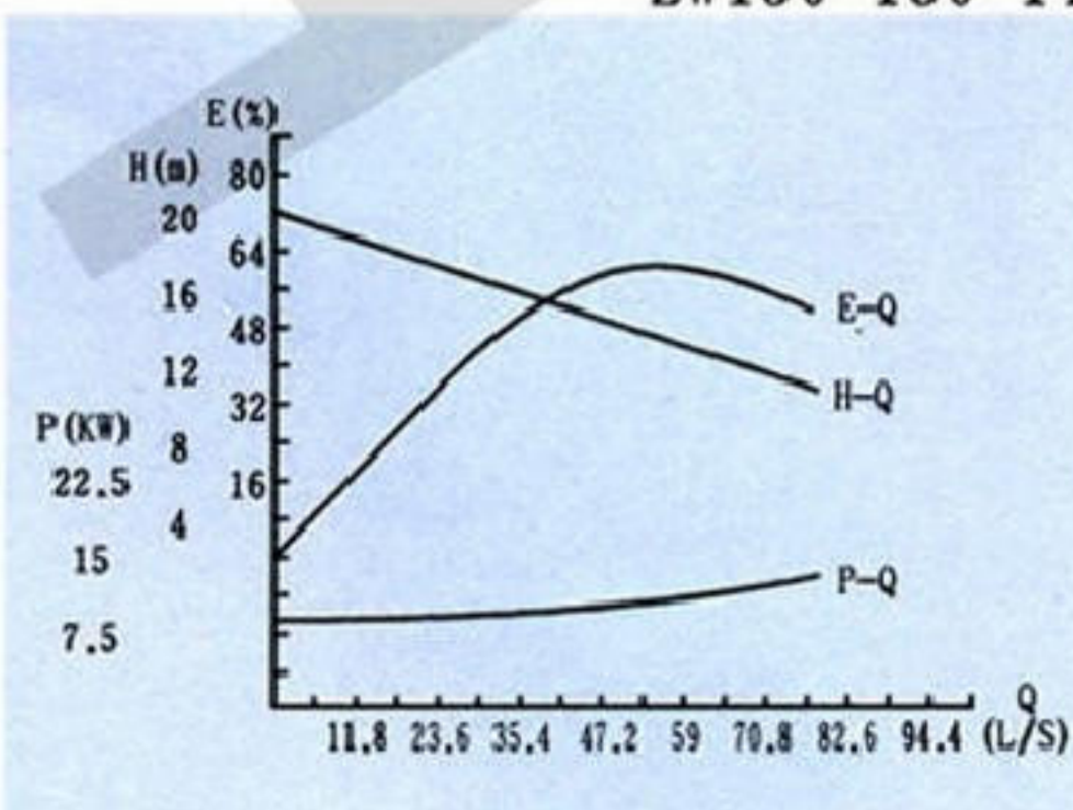
ZW150-180-14
