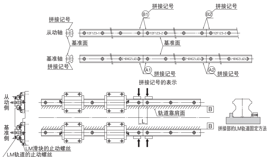
图4 拼接使用
