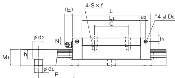
SVS-R型
