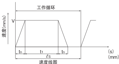
图8 使用条件
