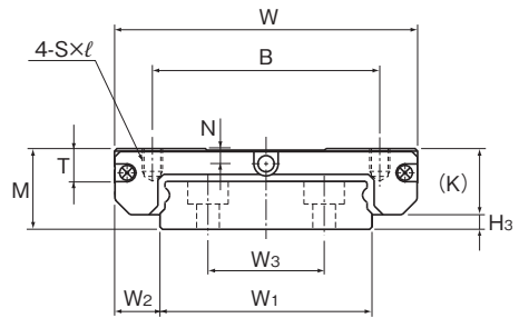
SRS15WM/WN型
