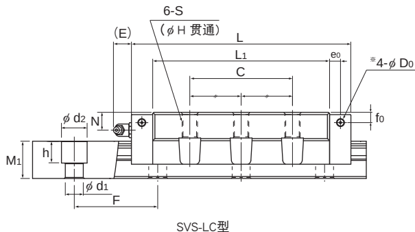
SVS-LC型
