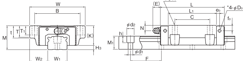
NR-B型
