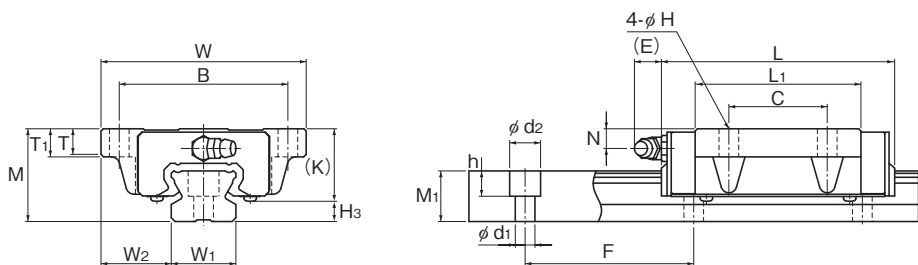
SR-M1TB型
