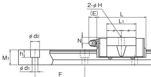
SR-M1SB型
