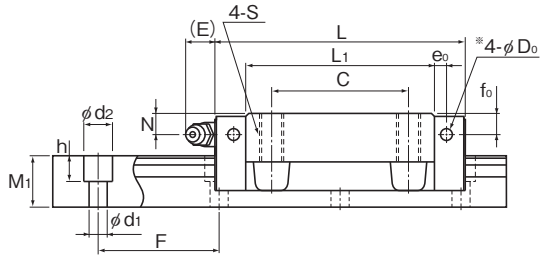
NRS-A型
