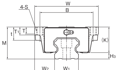
HSR45~85A/LA型
