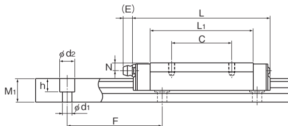
RSR15、20VM/N型
