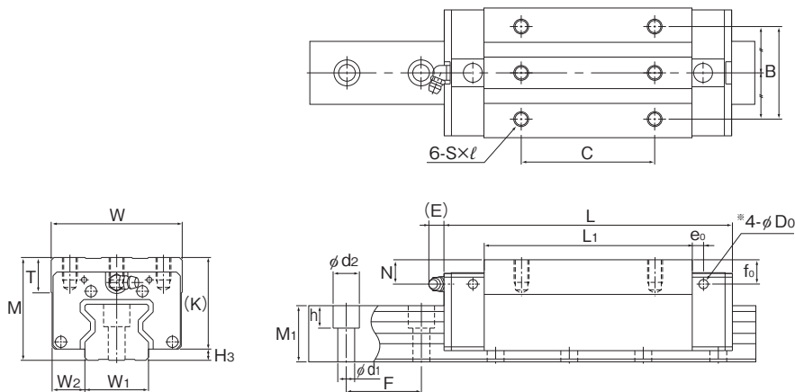
SRG25~65LR/LV型
