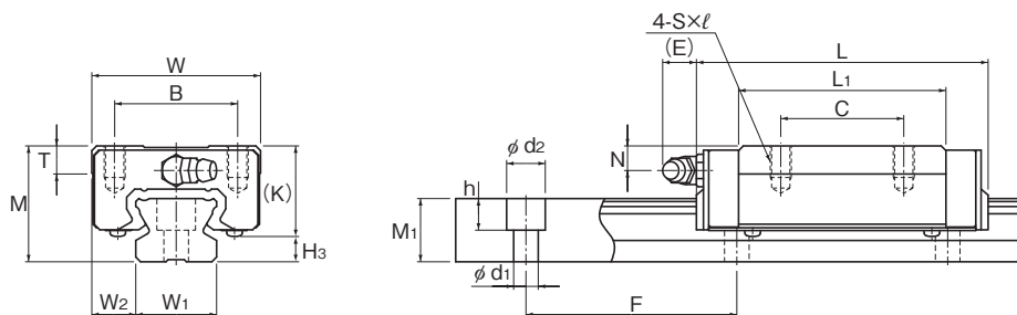
SR-M1W型
