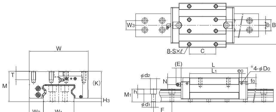
SRW70~100LR型
