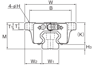
HSR20M1B/M1LB型
