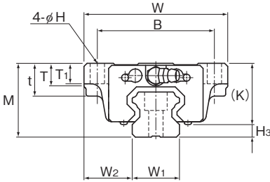
HSR15、25~35M1B/M1LB型
