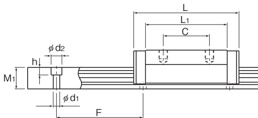
SHW27~50CR型
