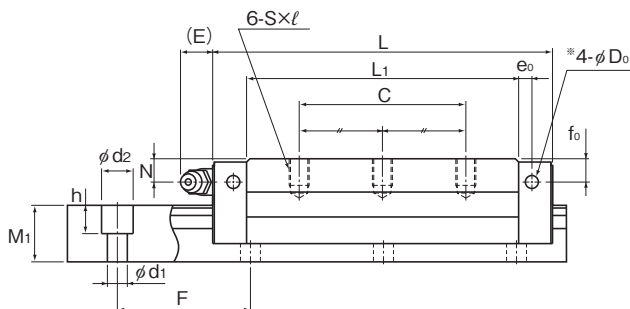
NR-LR型
