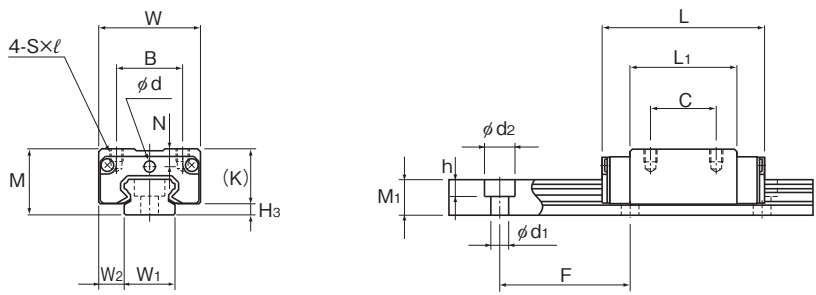
HSR8、10RM型
