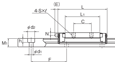
RSR15WZM型
