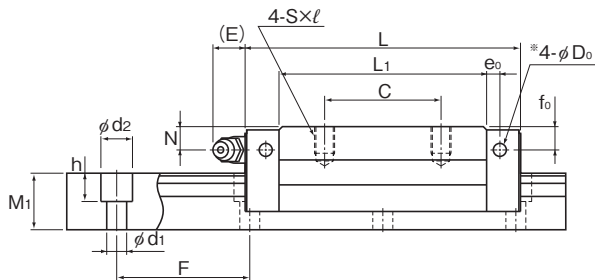
NR-R型
