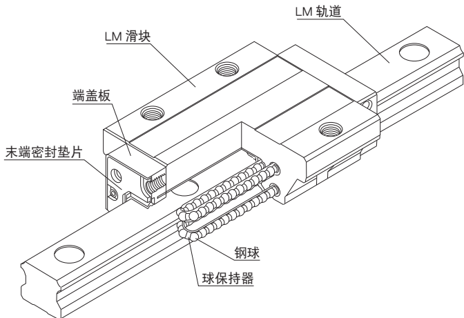
图1 球保持器型LM滚动导轨SHS型的结构图
