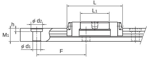
SRS5M型
