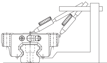
图11 行走平行度
