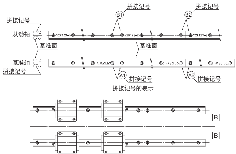
图23 拼接使用
