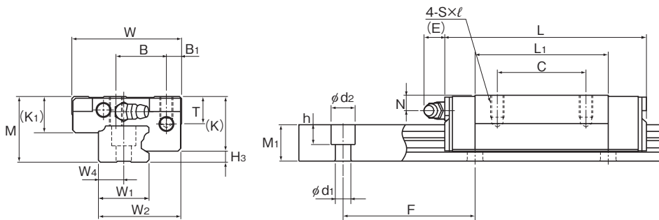
GSR20~35T型、GSR20,25V型
