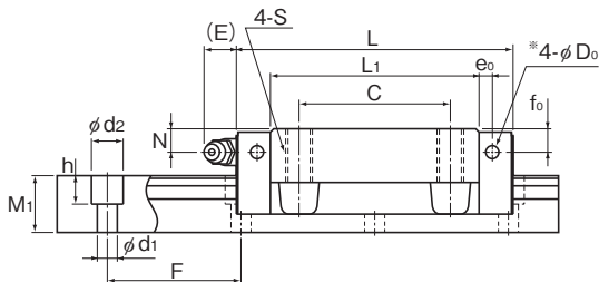
NR-A型
