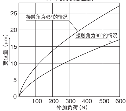
接触角不同时的负荷和变变量 ( D_a=6.35\text{mm} ) (单个钢球的变变量)
