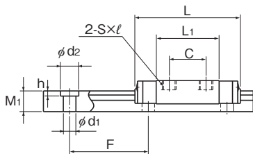
RSR5N型
