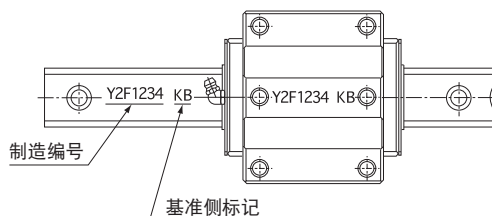
图16 基准侧的LM轨道
