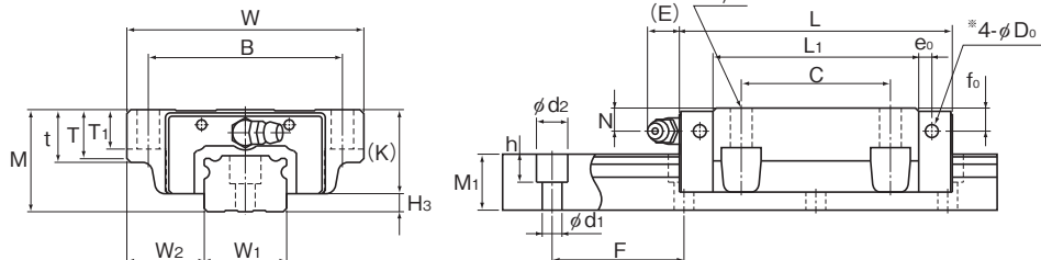
NRS-B型
