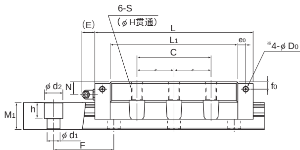
SVR-LC型
