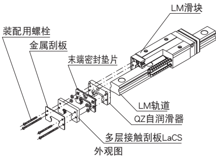
外观图
