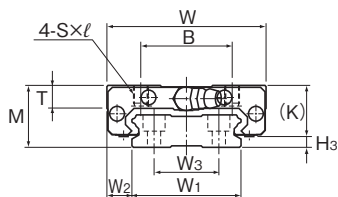
HRW17、21CR/CRM型
