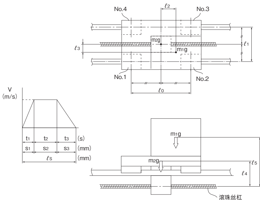
图12 使用条件
