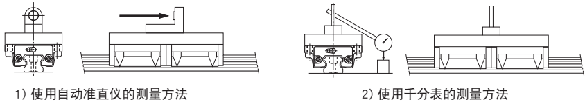
图35 安装后的精度测量方法
