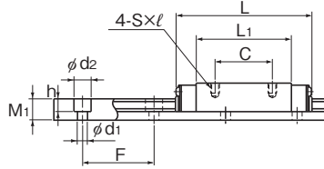
RSR7~12N/7M/9KM/12VM型
