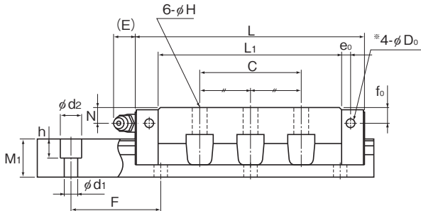
NR-LB型
