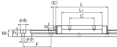
RSR15WV/WVM/WN型
