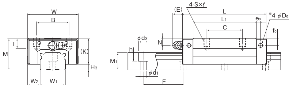
NRS-R型
