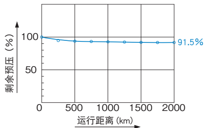
图7 运行距离与预压剩余率
