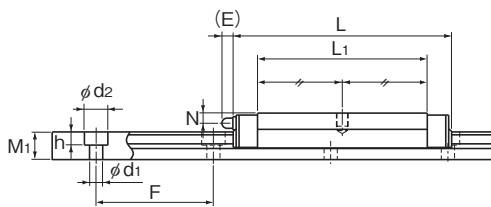
RSR5WTM/WTN型
