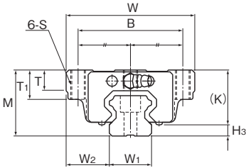
HSR20~35CA/HA/CAM/HAM型
