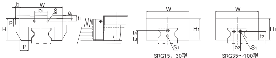
SRG15、30型
