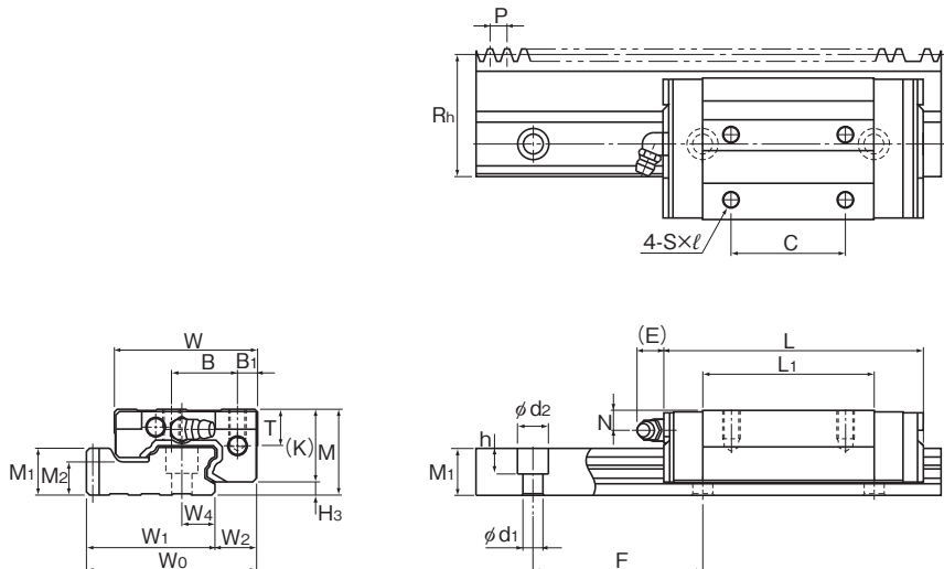
GSR-T-R型
