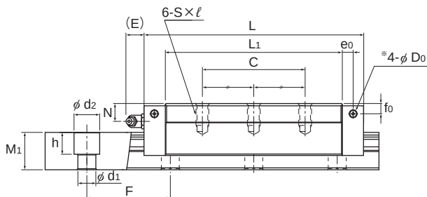
SVR-LR型
