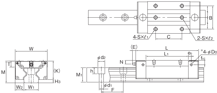
SRG15、20V/LV型
