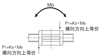
图4 M_B 力矩的等价系数
