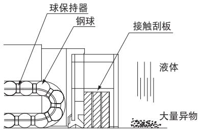
结构图
