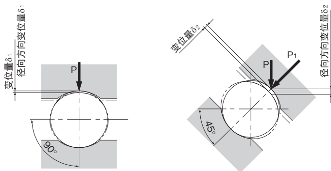
图3 径向载荷下的变变量
