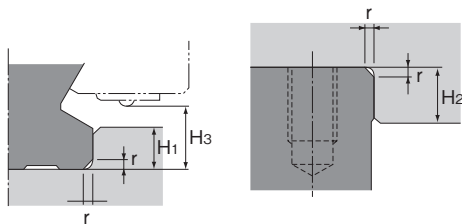
LM轨道的靠边
