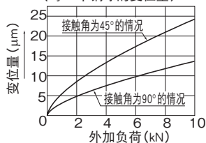
图2 径向载荷和变位置(通常间隙、无预压)
