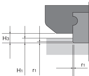
LM轨道的肩部
