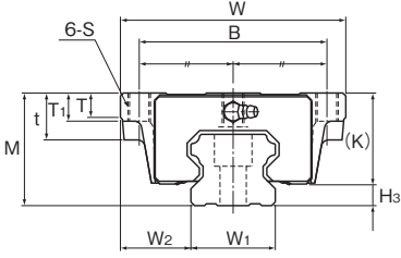
HSR45~85CA/HA型
