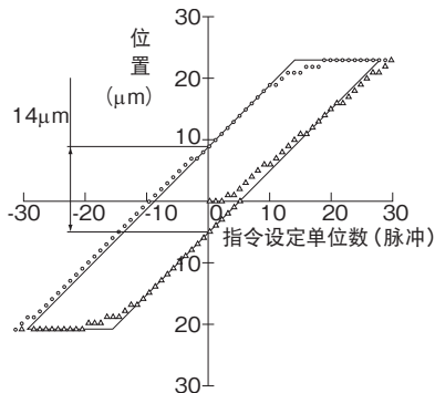
方滑板+贴塑导轨
