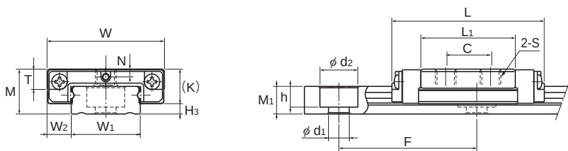
SRS5WM型
