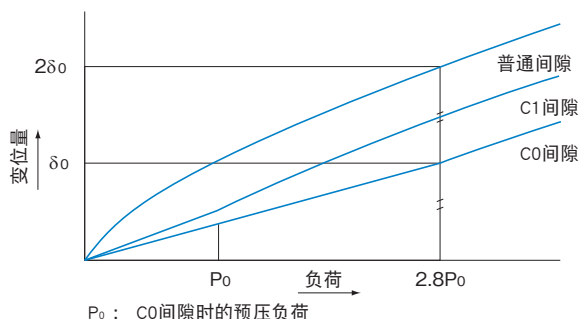
图14 刚性数据
