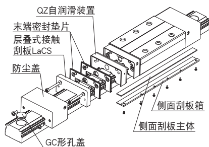
外观图(例：QZTTHHY型的情况)
