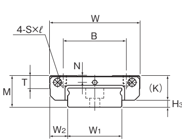
SRS7WM/9、12WM/WN型
