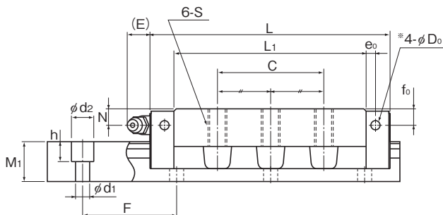
NRS-LA型
