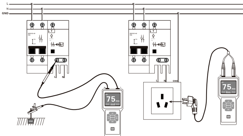
单相电路漏电保护器测试示意图
