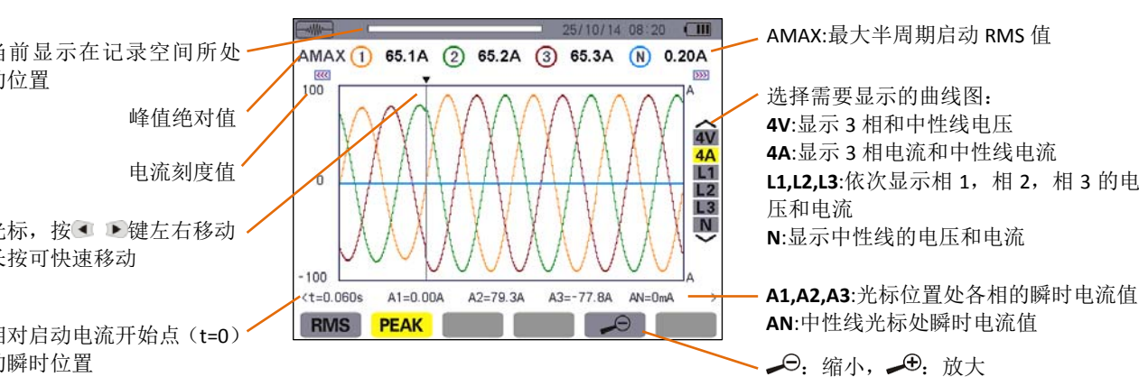
图 6-11 4A 峰值显示屏幕
