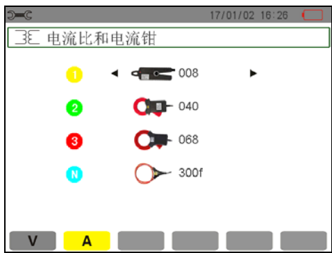
图 5-8 电流钳及变比设置菜单
