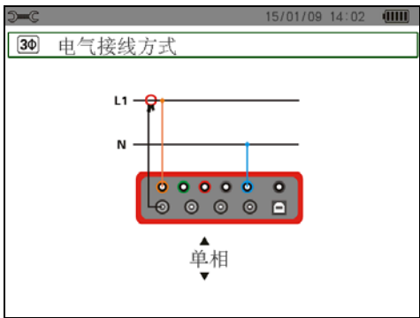
图 4-4 单相连接
