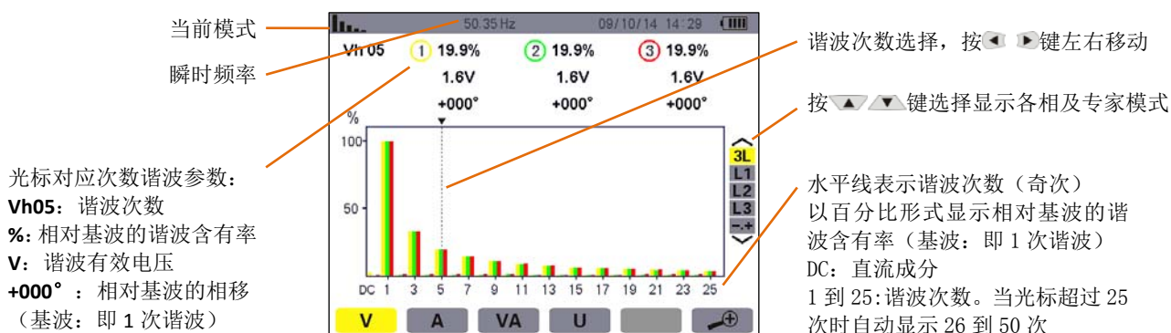
图 7-2 相电压谐波 3L 显示
