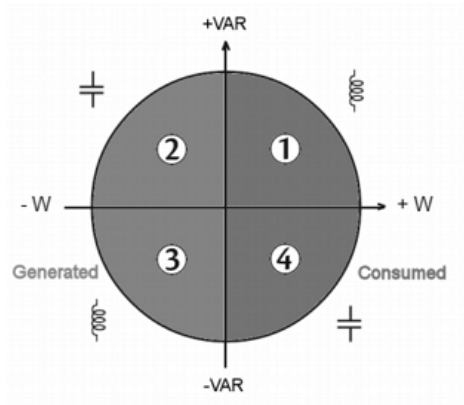
图 17-3 功率电能象限图
