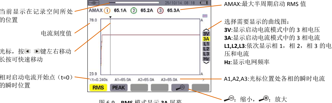
图 6-9 RMS 模式显示 3A 屏幕
