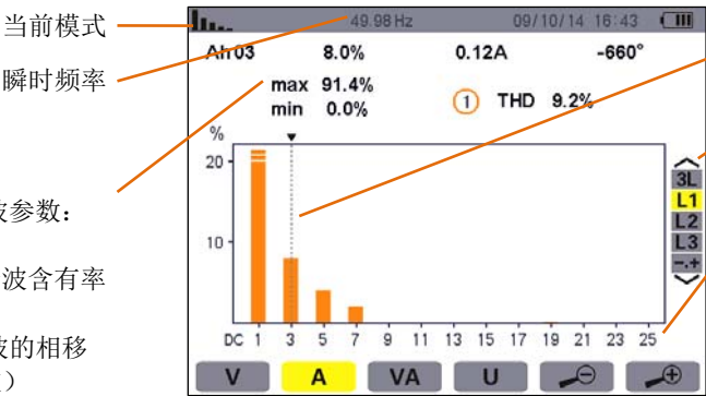
图 7-5 电流谐波 L1 显示
