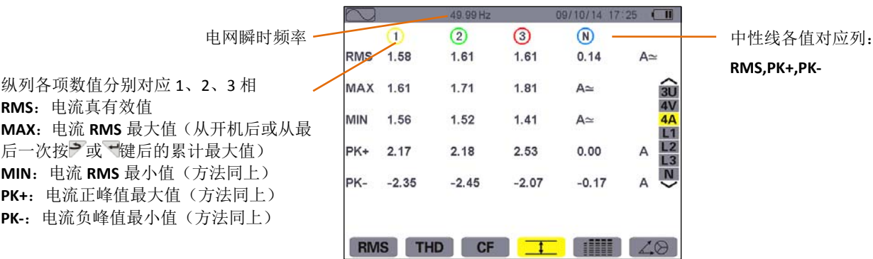
图 8-14 4A 下 Max-Min.显示屏幕
