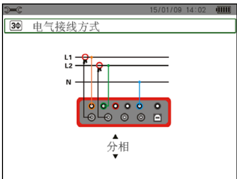
图 4-5 分相连接
