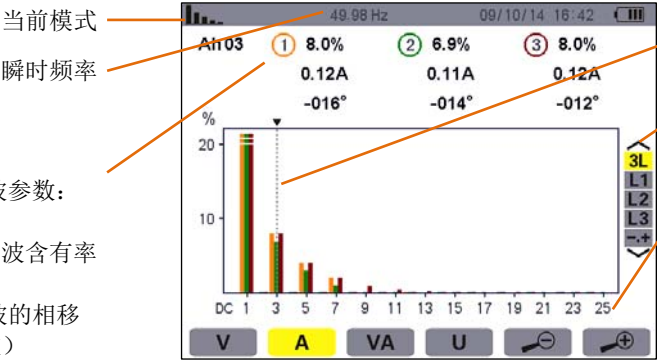
图 7-4 电流谐波 3L 显示
