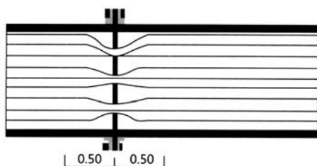
平衡流量计直管段要求低
