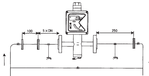
XTLZ3 安装图
