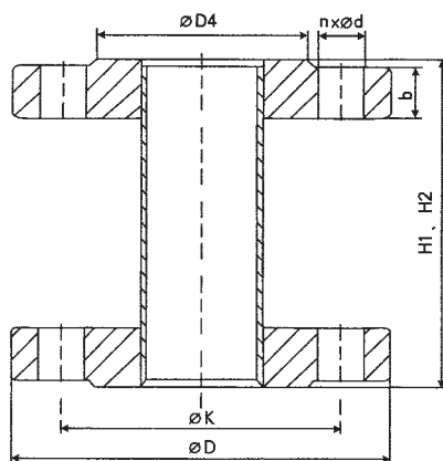
直管段
