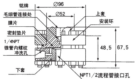
(1199) RTW 型螺纹安装式远传装置 (最大工作压力 10MPa) 外型尺寸图
