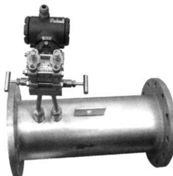
V 锥流量计 (一体型)
