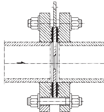
限流孔板
