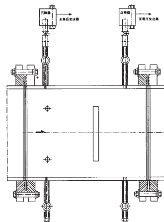
环形孔板
