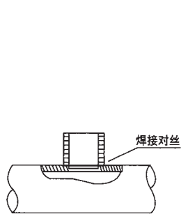
图二焊接对丝
