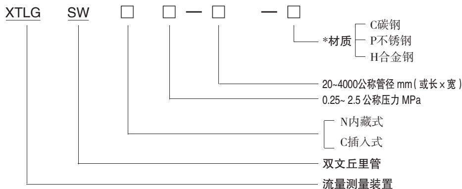
插入式双文丘里管
