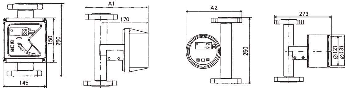
XTLZ0安装 M2 指标器 (M1 指标器同)
