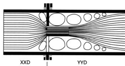
孔板流量计直管段要求很长
