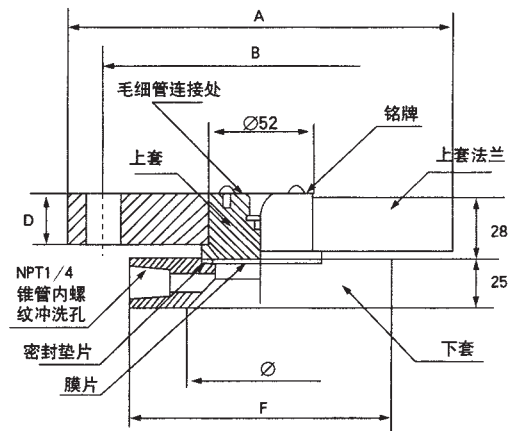
(1199) RTW 型螺纹安装式远传装置 (最大工作压力 10MPa) 外型尺寸图
