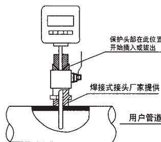
图三插入和拔出保护管
