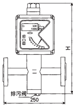
XTLZ3 ( DN50 )
