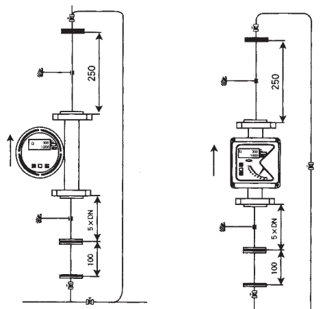
XT LZ0安装图
