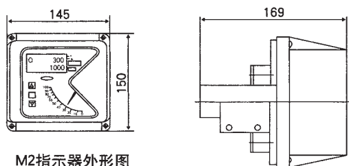
M2指示器外形图
