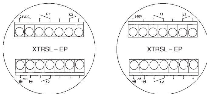
图三 一体化结构 接线端子外接线图
