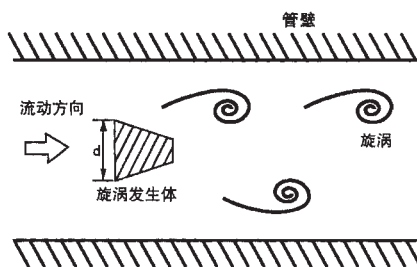
图 1 卡曼涡街
