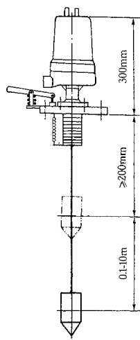
UQK-66□C型
