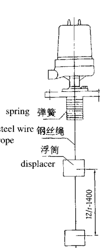
UQK-66□T型
