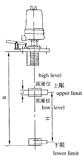
UQK-66□T型
