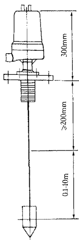
UQK-66□C型
