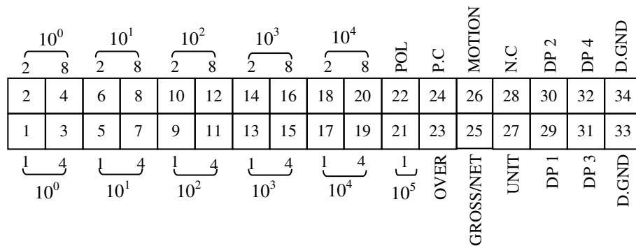
BCD 插 座
