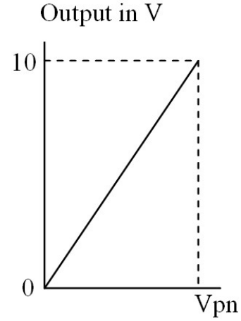
(图 3: 0-10VDC 输出)
