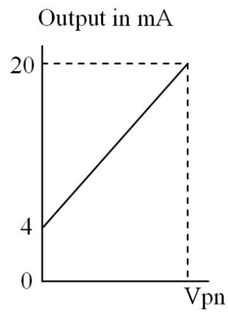
(图 1: 4-20mA 输出)
